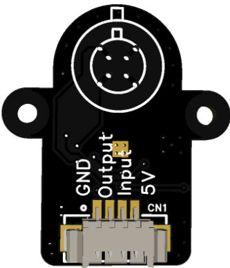
图 8. 模组示意图
