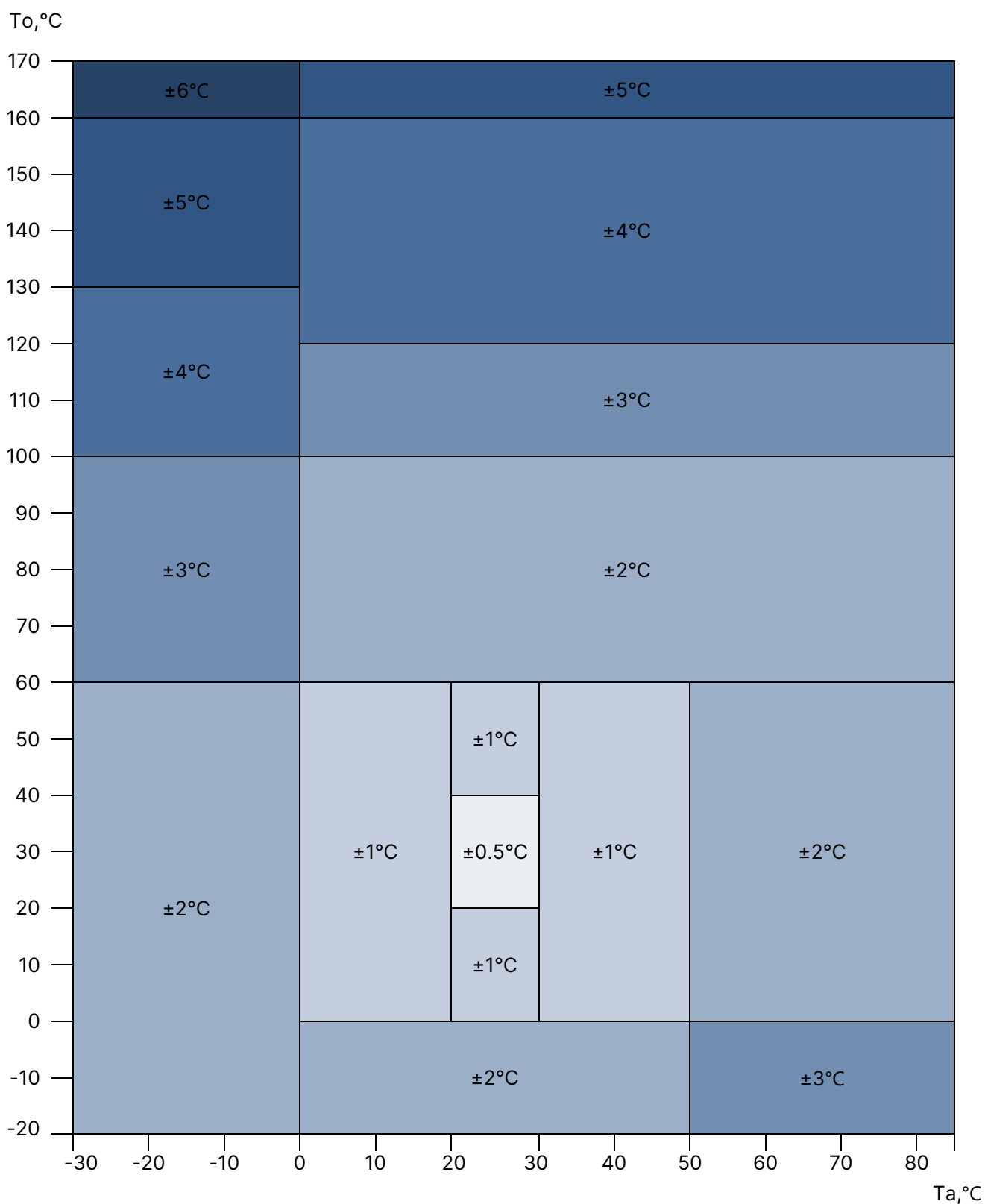
图 3. LMW-MT0/WD1 ( T_a, T_o ) 的标准精度
