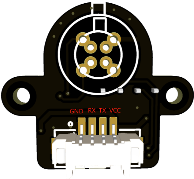
图 8. 模组示意图
