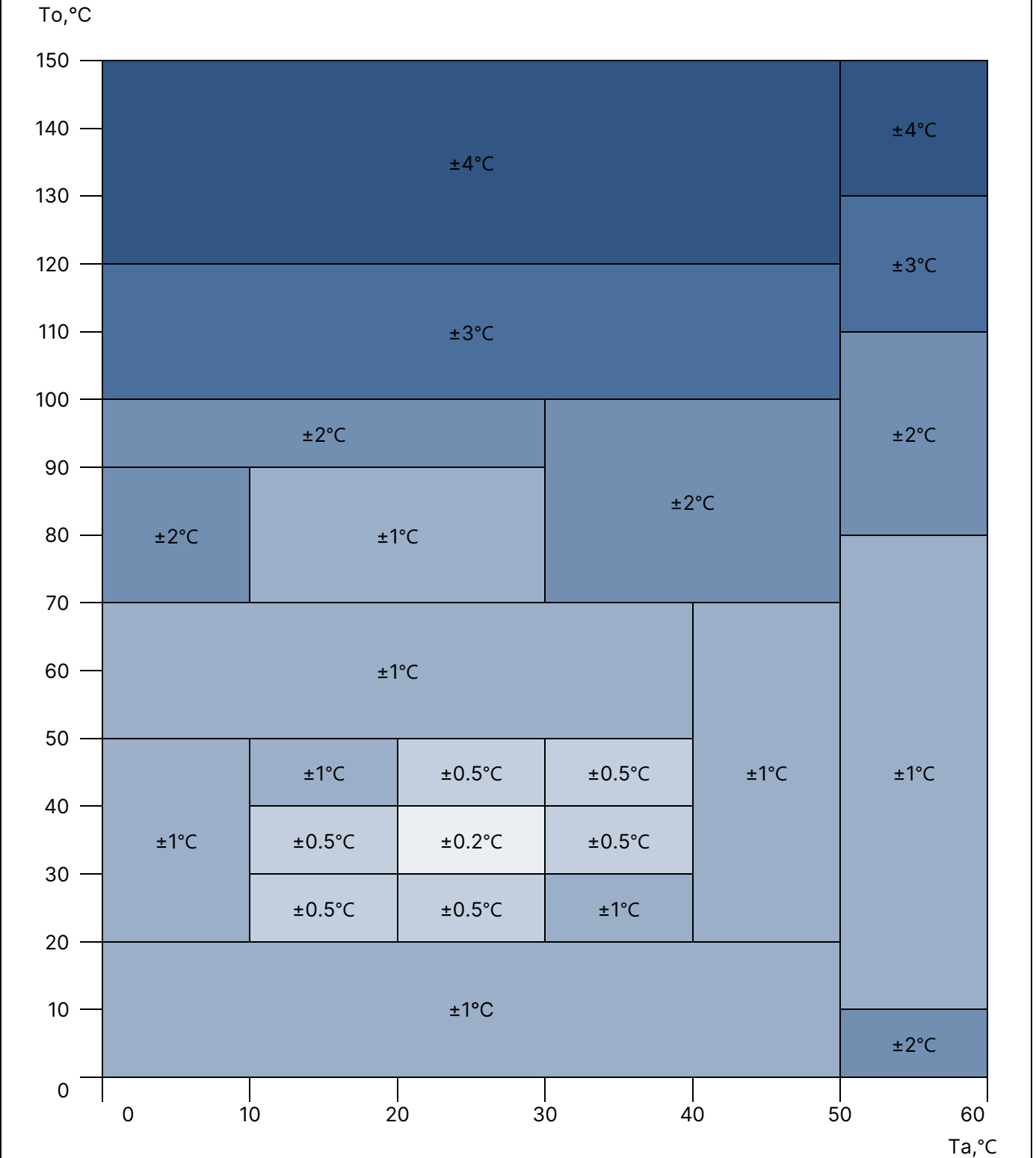
图 4. LMW-MT1/FD1C (Ta, To) 的标准精度
