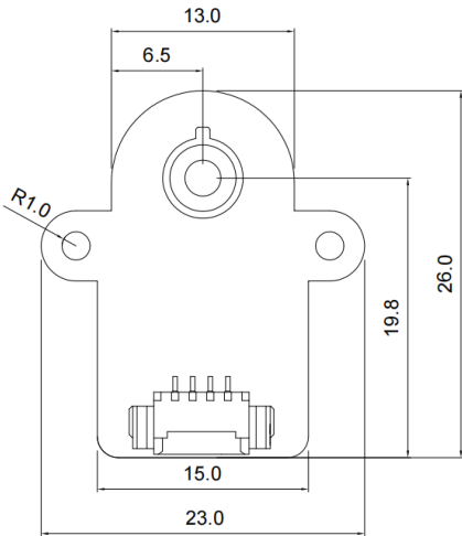
图 9. 模组板框尺寸图
