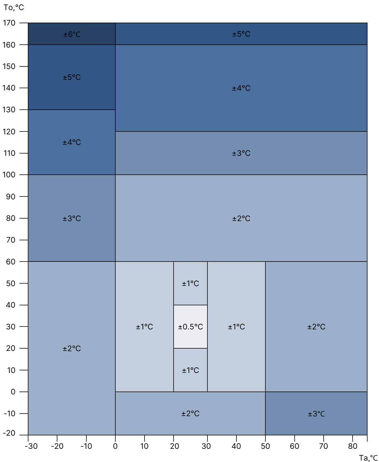
图 3. LMW-MT4/WD5I ( T_a, T_o ) 的标准精度
