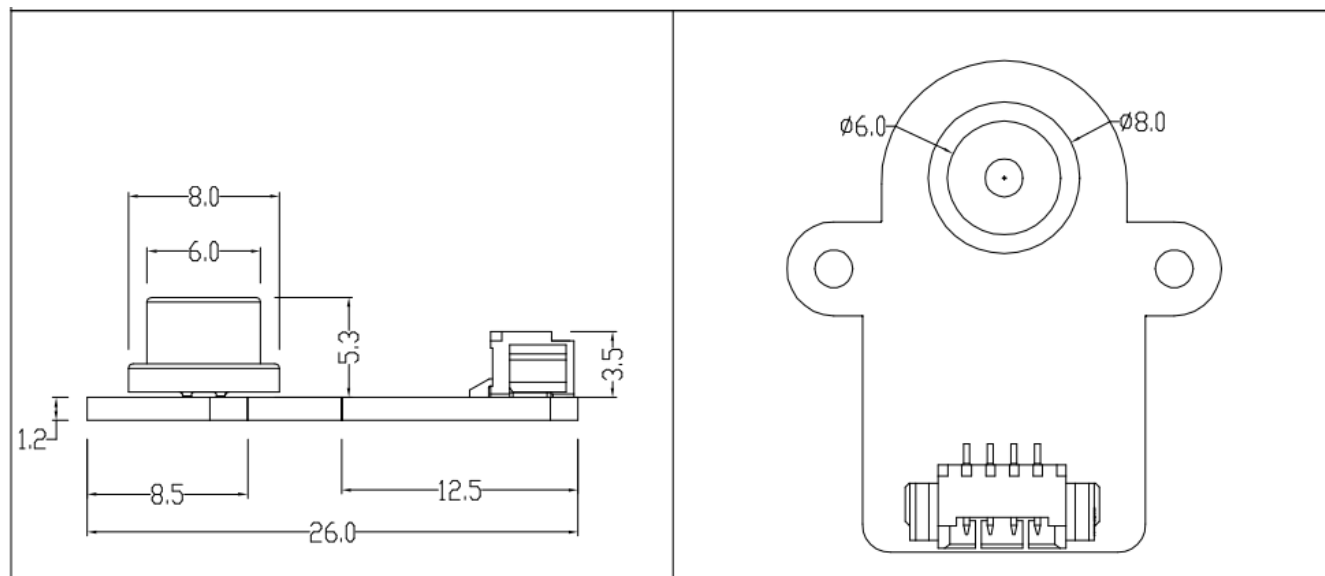
图 10. 模组外形尺寸图
