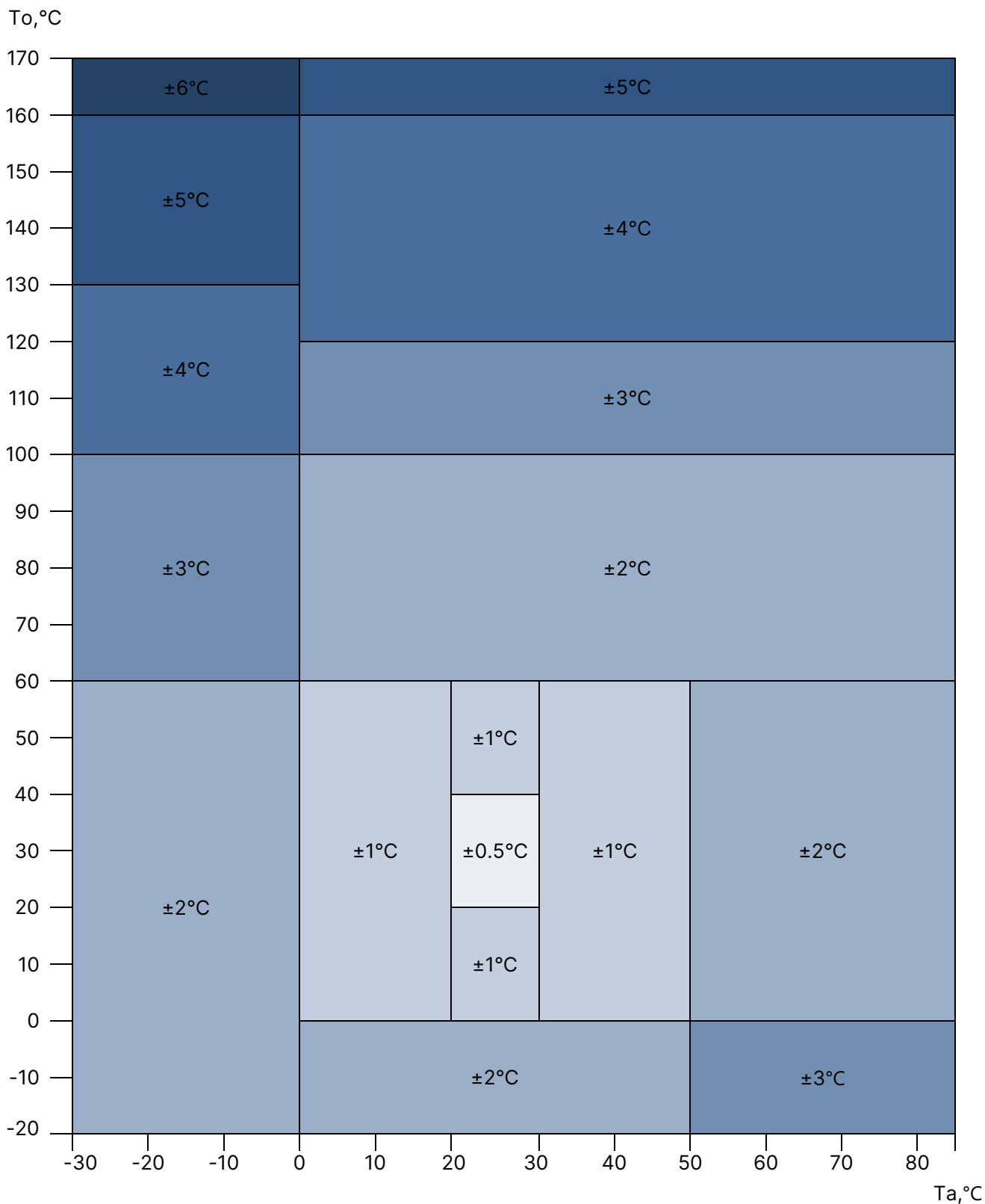
图 3. LMW-MT0/WD4I (Ta, To) 的标准精度
