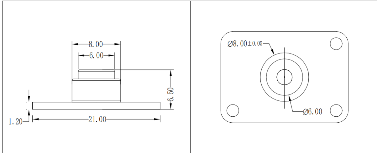
图 10. 模组外形尺寸图
