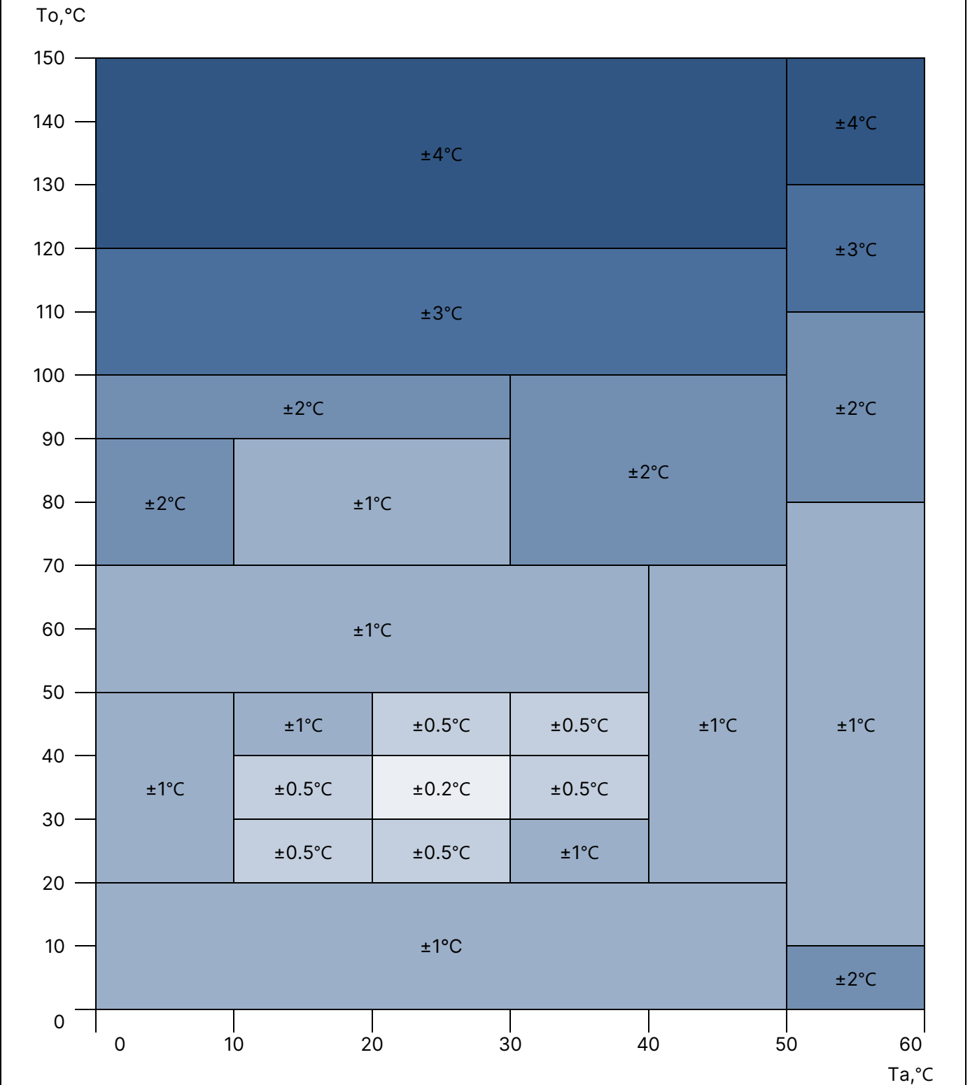
图 4. LMW-MT5/FD1C (Ta, To) 的标准精度
