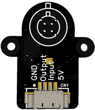
图 8. 模组示意图
