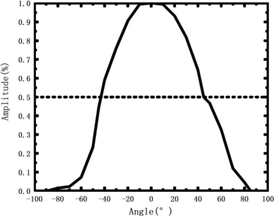
图 2.传感器的视场角
