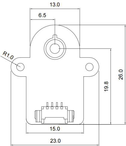
图 9. 模组板框尺寸图
