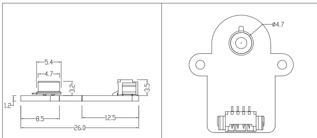
图 10. 模组外形尺寸图
