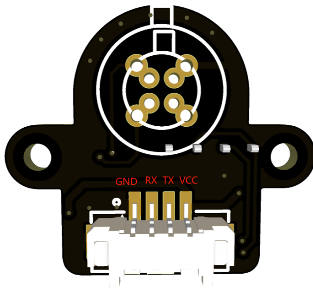
图 8. 模组示意图
