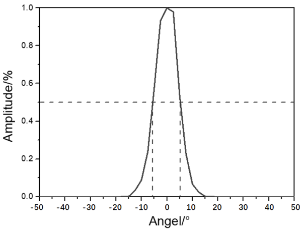
图 2.传感器的视场角
