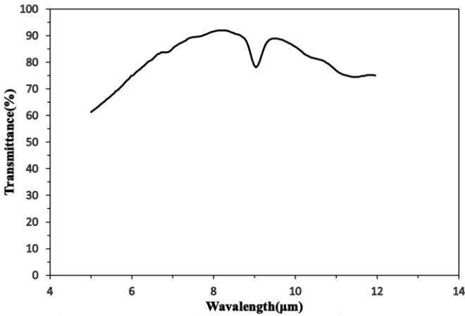
图 1. 滤光片的透过光谱
