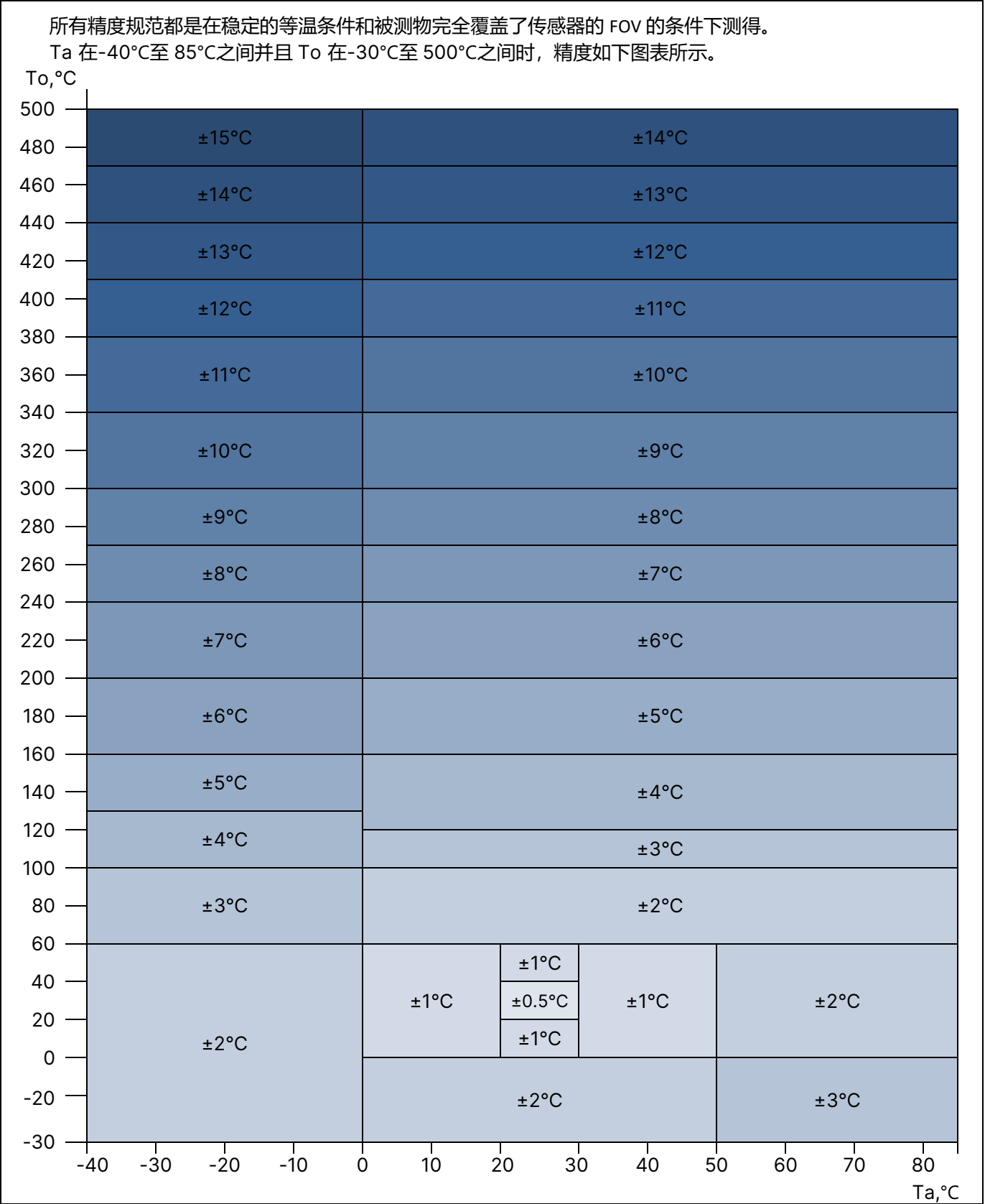
图 3. LMW-MT0/FD1I (Ta, To) 的标准精度
