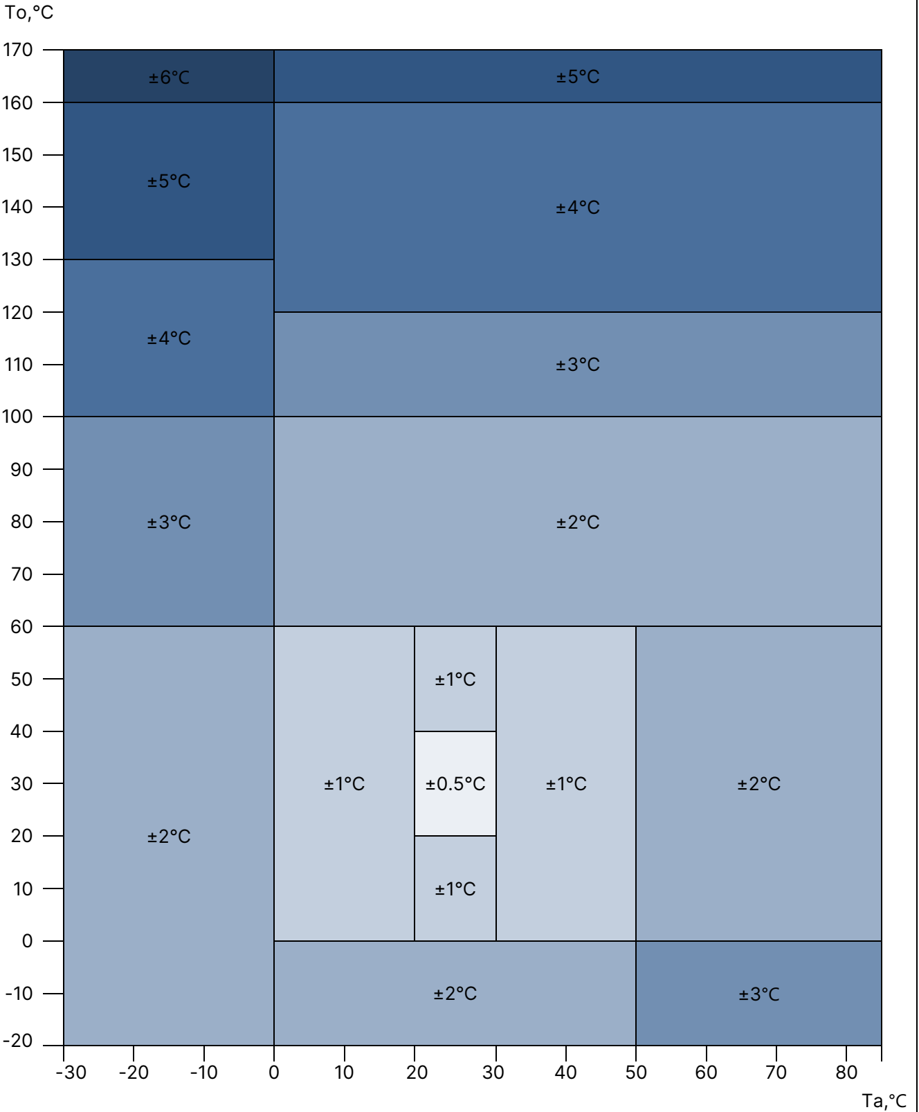
图 3. LMW-MT1/WD1I (Ta, To) 的标准精度
