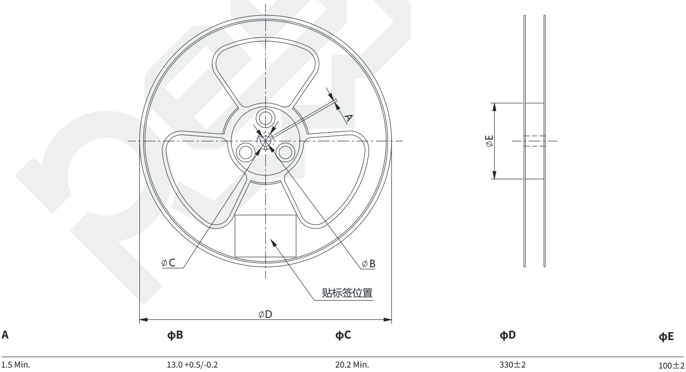
卡盘尺寸图
