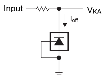
图 22 关断器的测试电路
