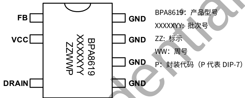
图 2. DIP-7 管脚封装图
