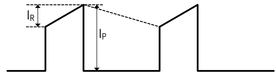
图13. 连续模式下初级电流波形
