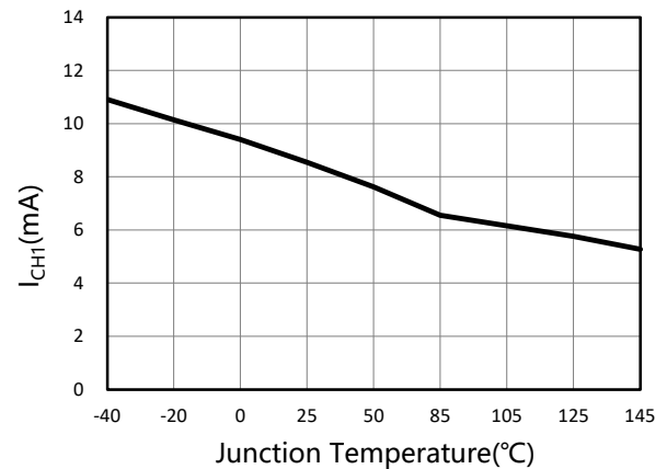
图 22. I CH1 vs. Temperature
