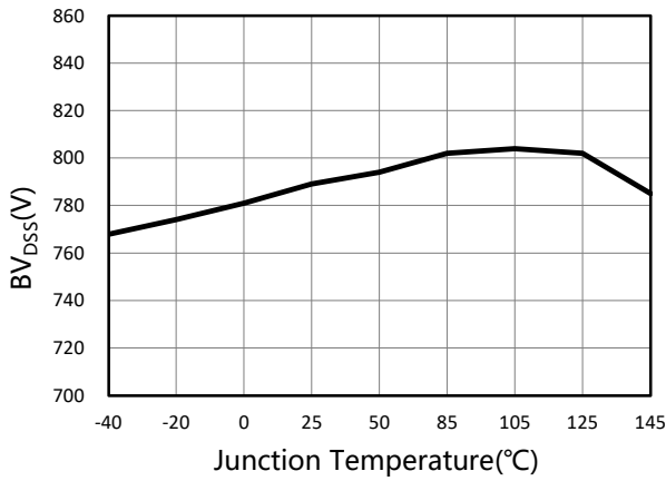
图 17. BV DSS vs. Temperature
