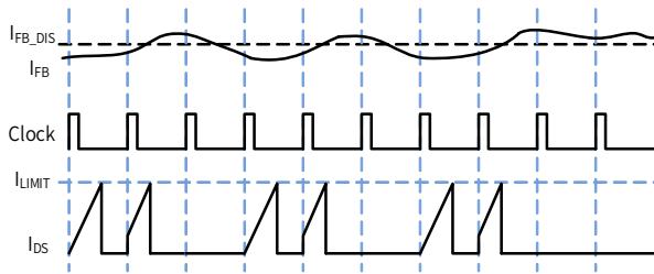
图 8. 脉冲数控制
