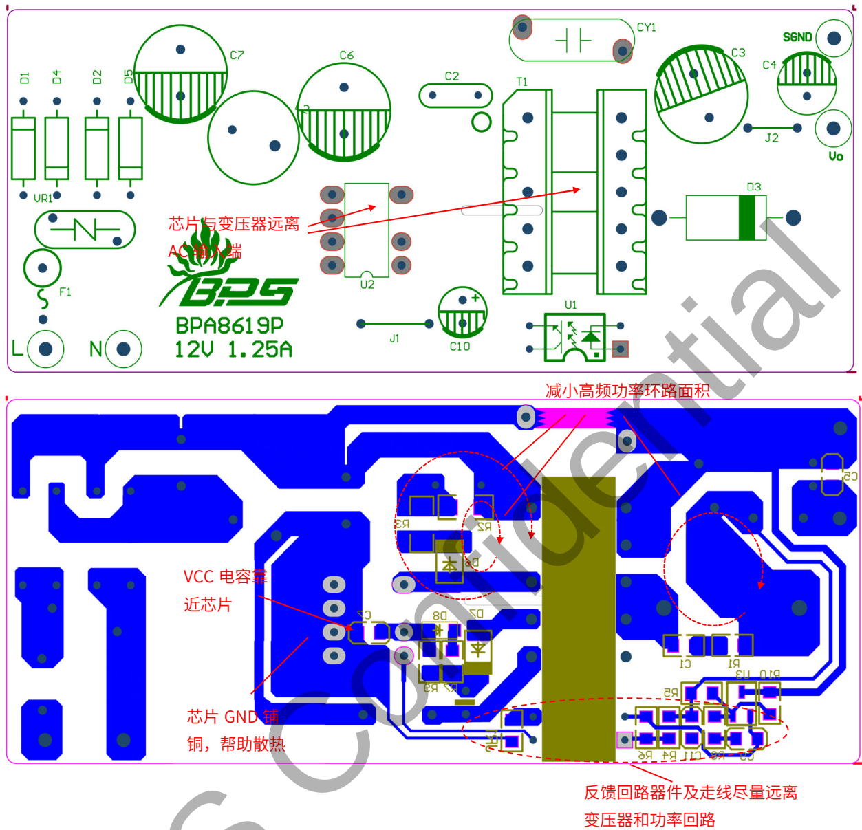
图 16. PCB Layout 建议
