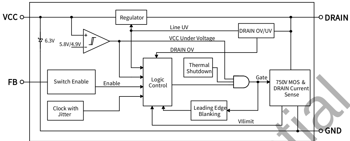
图 3. BPA8619P 内部框图
