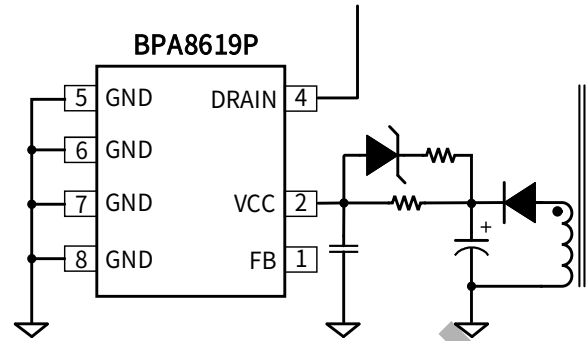
图 6. VCC 引脚实现输出电压保护
