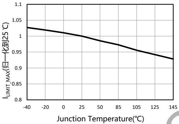
图 19. I LIMIT_MAX vs. Temperature
