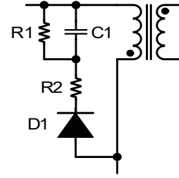
图15. RCD钳位电路
