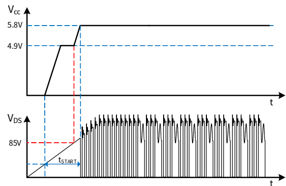
图 4. 高压启动时序
