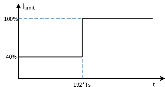
图 7. BPA8619P 软启动过程
