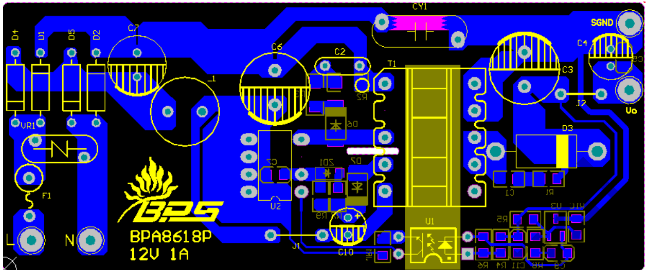
图 18. BPA8618P 设计实例 PCB Layout (单面板)
