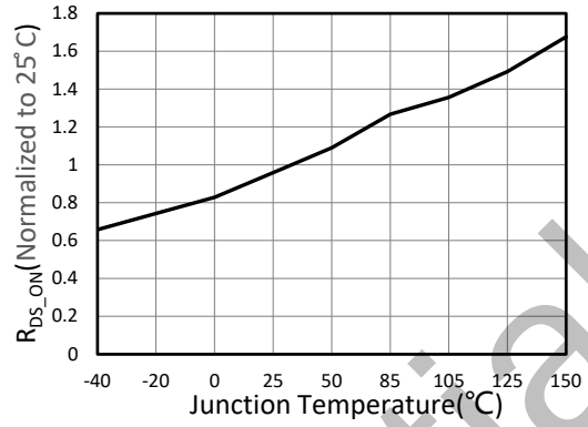
图 20. R DS_ON vs. Temperature
