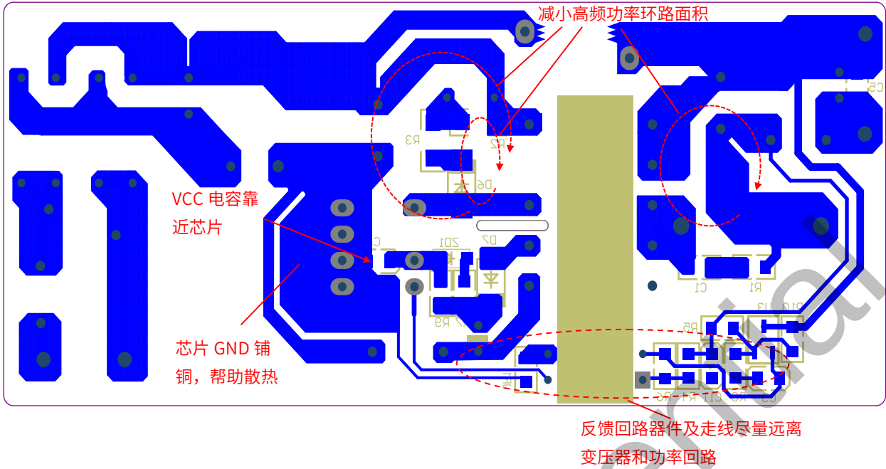
图 16. PCB Layout 建议
