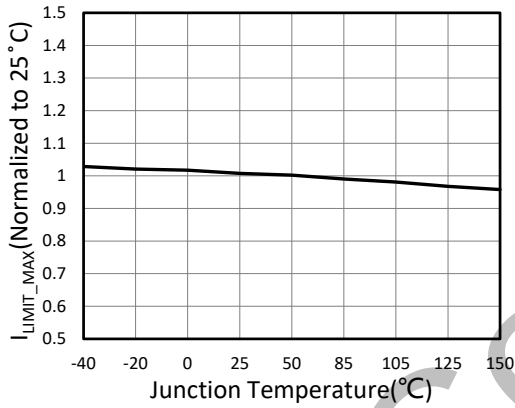
图 21. I LIMIT_MAX vs. Temperature
