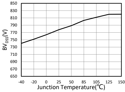
图 19. BV DSS vs. Temperature
