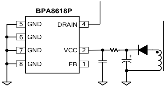
图14. 辅助绕组供电电路
