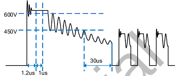
图 11. 工作过程中输入过压保护
