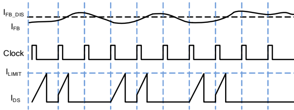
图 8. 脉冲数控制
