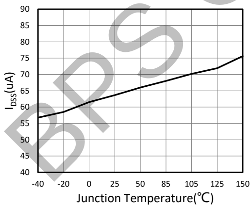
图 23. I DSS vs. Temperature
