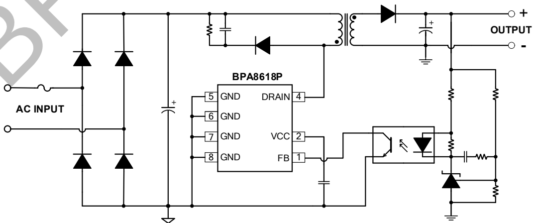
图 1. BPA8618P 典型反激应用电路
