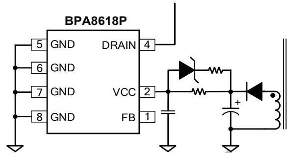
图 6. VCC 引脚实现输出电压保护
