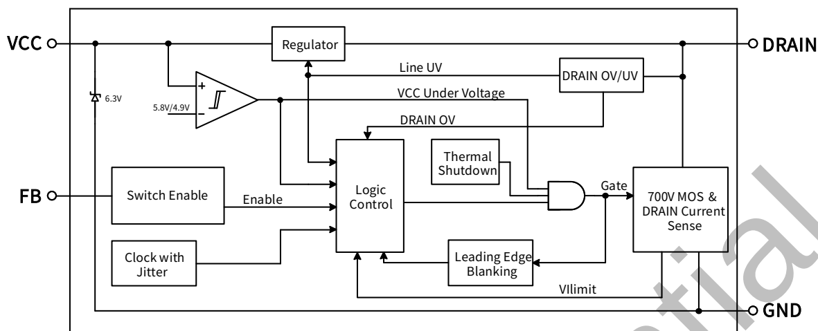
图 3. BPA8618P 内部框图
