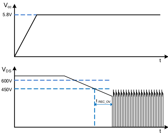
图 10. 开机时输入过压
