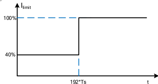
图 7. BPA8618P 软启动过程
