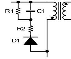
图15. RCD钳位电路
