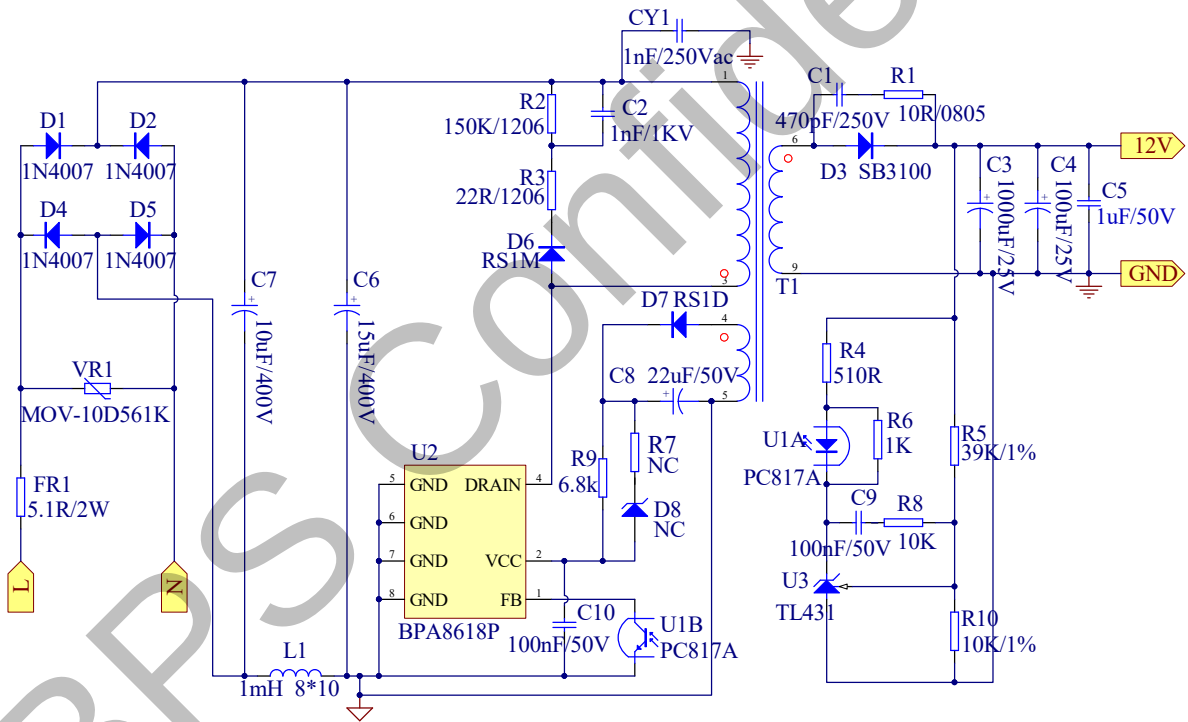
图 17. BPA8618P 设计实例电路图，85~265VAC 输入，12V/1A 输出
