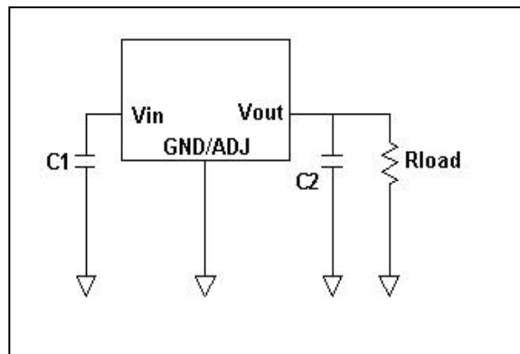
图 1 D1117 固定电压版本应用电路
