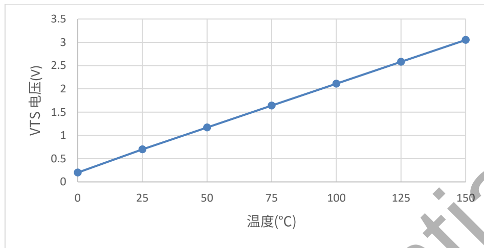
图 4.VTS 输出特性曲线
