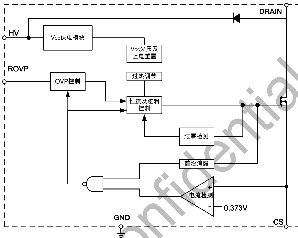
图 3 BP2891XJ 内部框图
