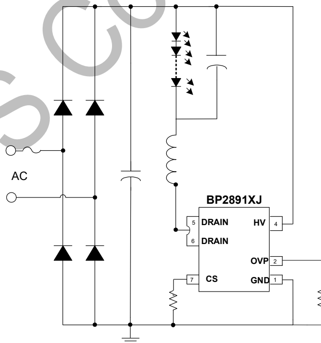
图 1 BP2891XJ 典型应用图
