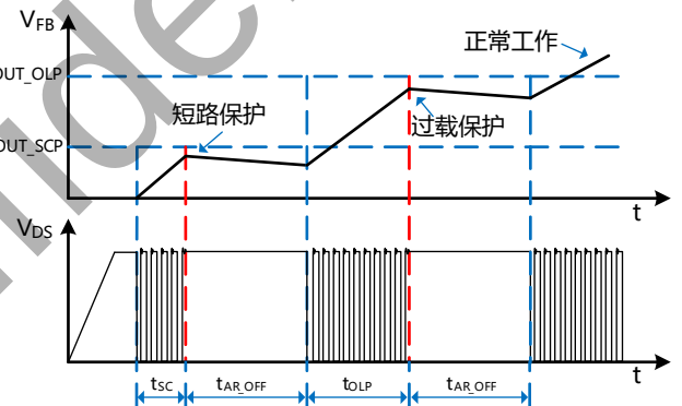
图 9. 过载保护工作模式
