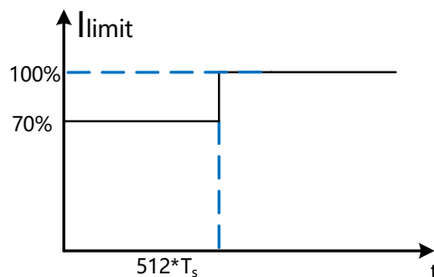
图 6. 软启动过程
