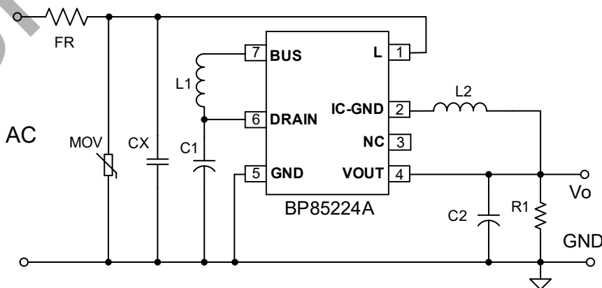
图 1. BP85224A 典型 Buck 应用电路
