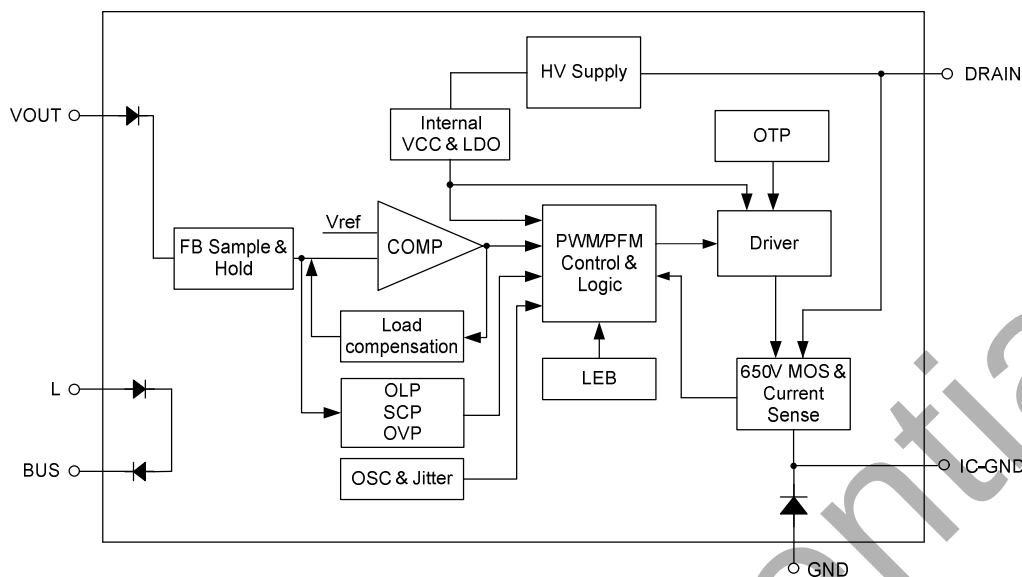
图 4. BP85224A 内部框图
