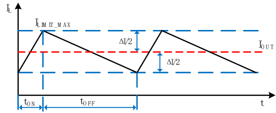
图 10. CCM 模式下的电感电流
