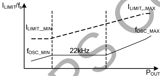
图 8. 控制模式
