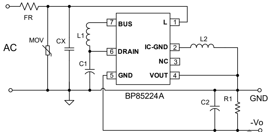
图 2. BP85224A 典型 Buck-Boost 应用电路
