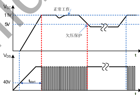
图 5. 高压启动与 VCC 欠压保护时序
