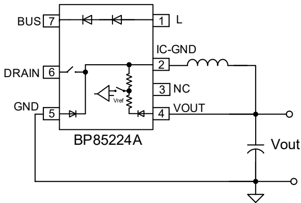
图 7. 输出电压采样示意图
