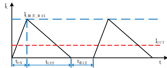
图 11. DCM 模式下的电感电流
