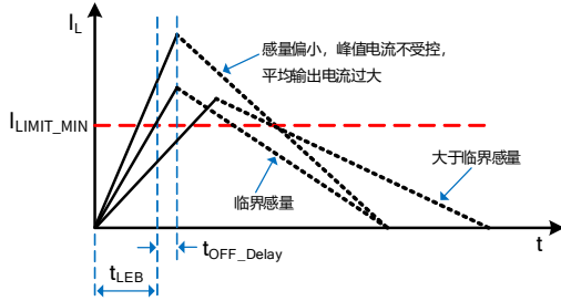
图 12. 空载下的电感电流
