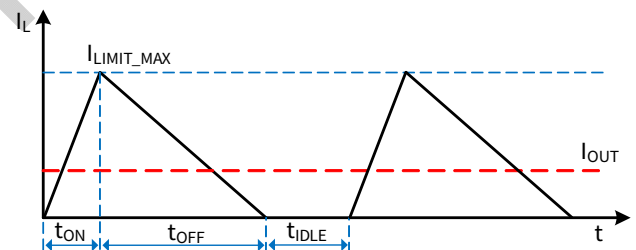
图 9. DCM 模式下的电感电流
