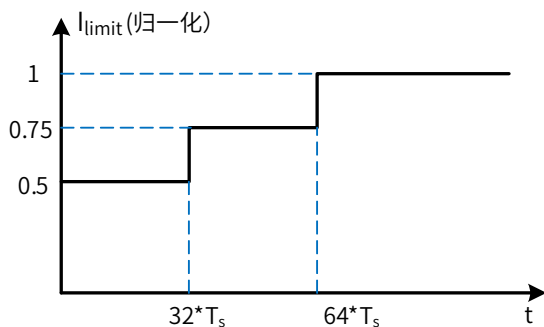
图 5. 软启动过程
