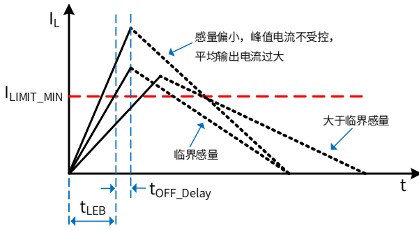
图 10. 空载下的电感电流
