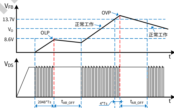
图 7. 过载保护、输出过压保护工作模式
