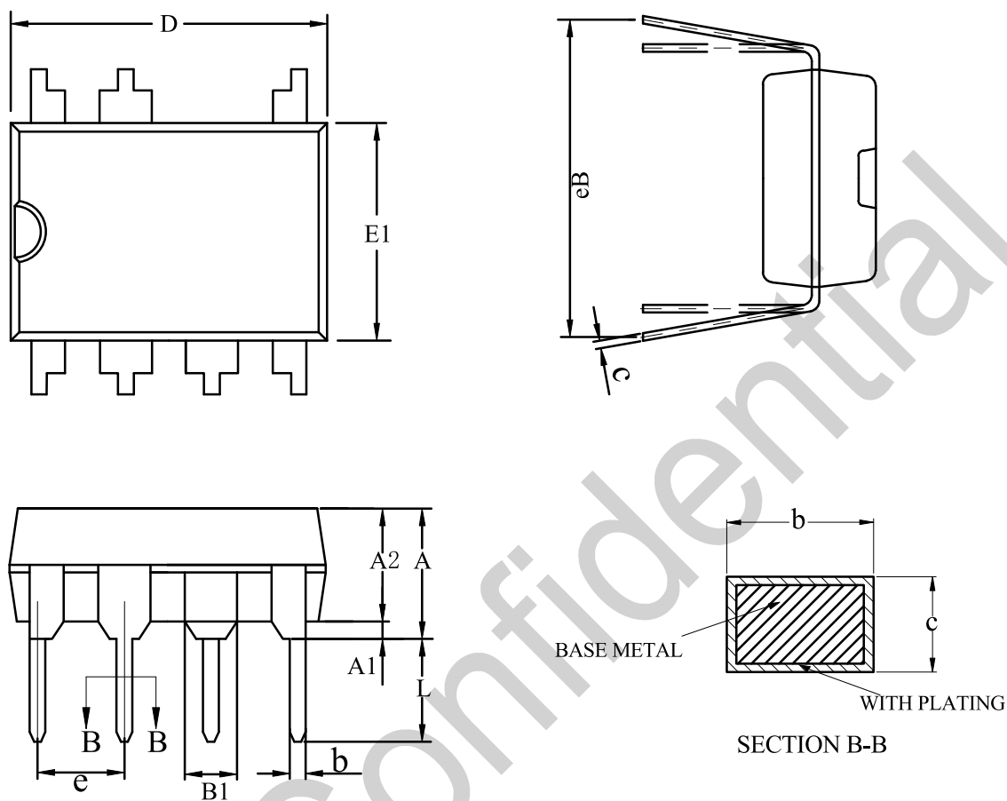
DIP-7 封装外形尺寸
