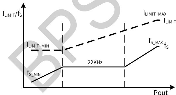
图 6. 控制模式
