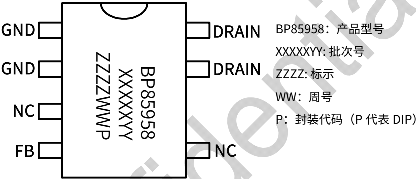
图 2. 管脚封装图
