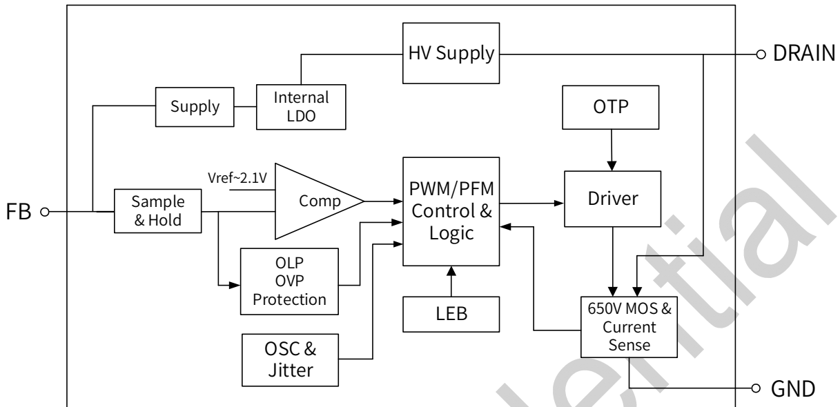
图 3. BP85958P 内部框图
