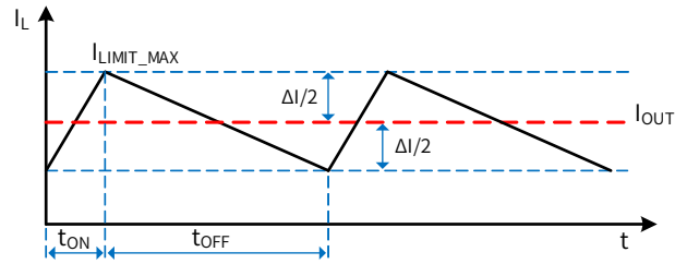
图 8. CCM 模式下的电感电流
