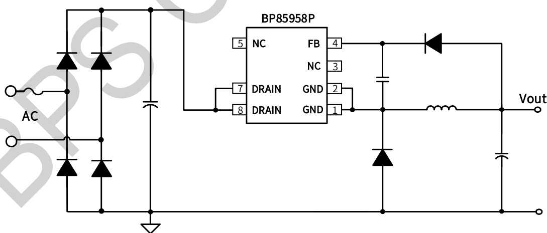
图 1. BP85958P 典型应用电路
