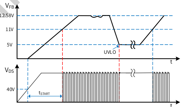
图 4. 高压启动与 FB 欠压保护时序
