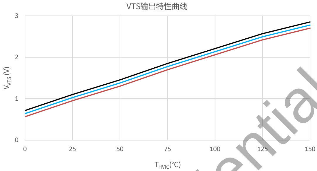
图 7. VTS 输出特性曲线
