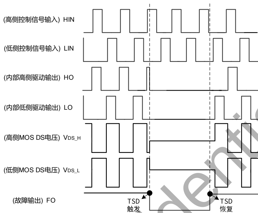
图 7. 热关断逻辑
