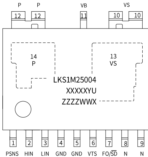
图 2. LKS1M25004U 管脚封装图
