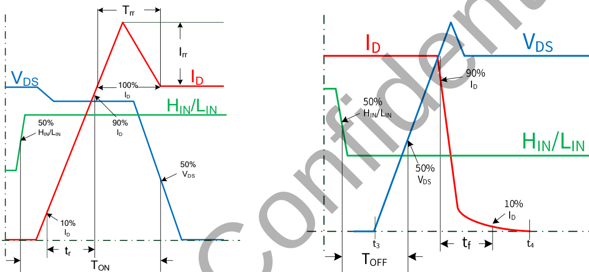
图 4.开关过程时间定义
