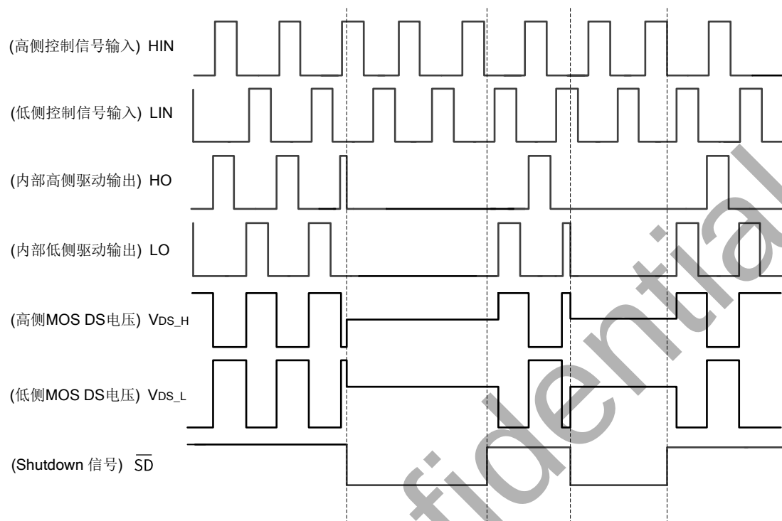
图 6. 外部关断控制逻辑
