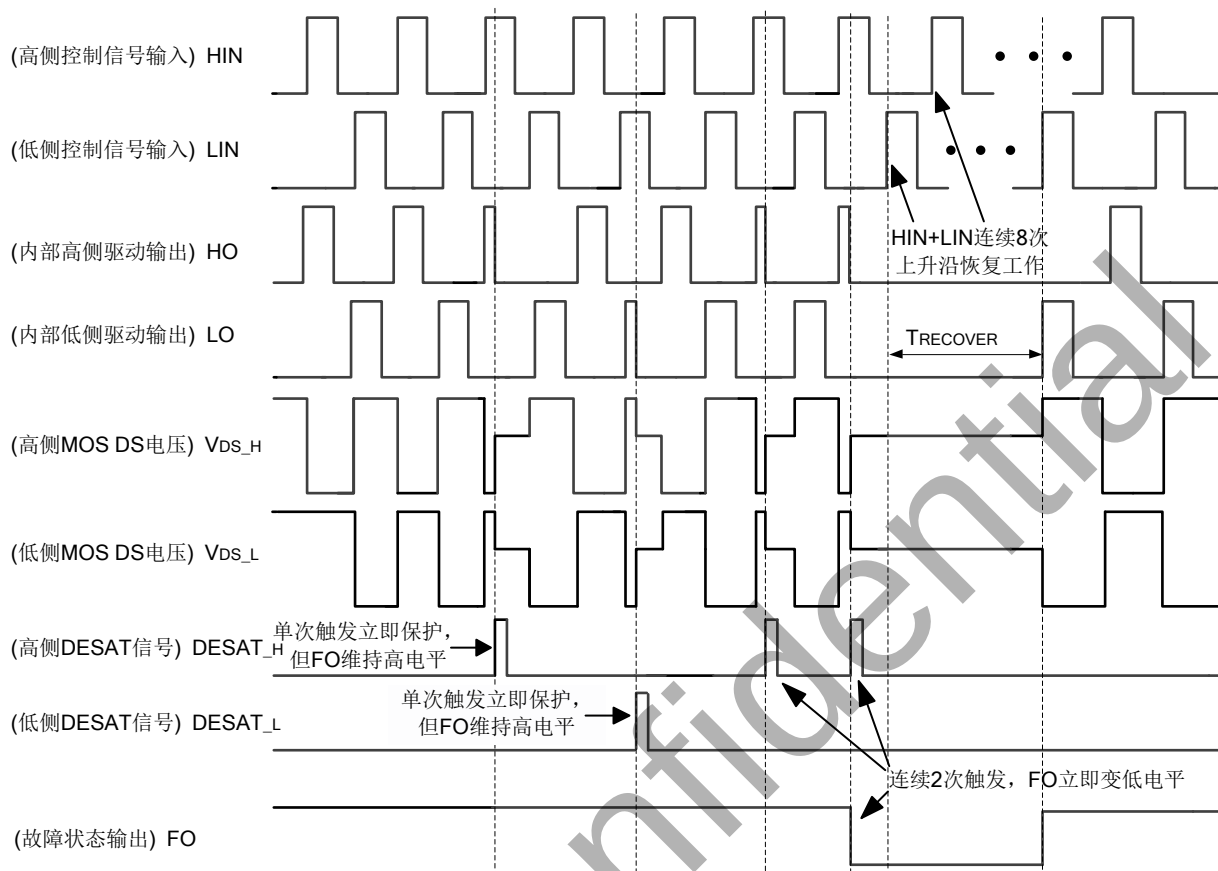
◆ 图 4. DESAT 保护功能
