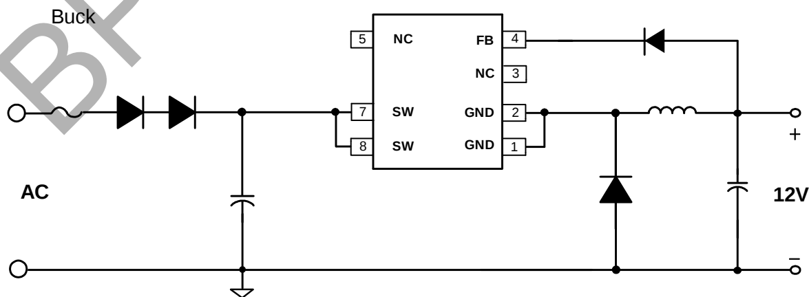
图 1. BP85956P 典型 Buck 应用电路
