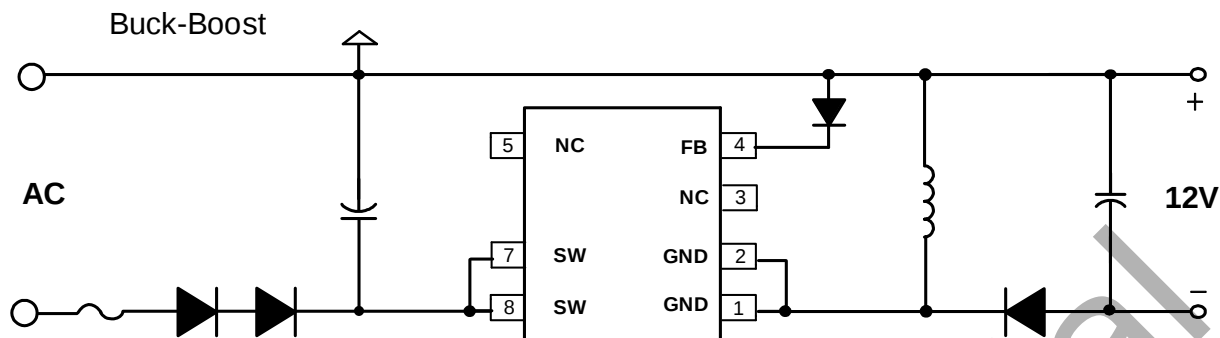
图 2. BP85956P 典型 Buck-boost 应用电路
