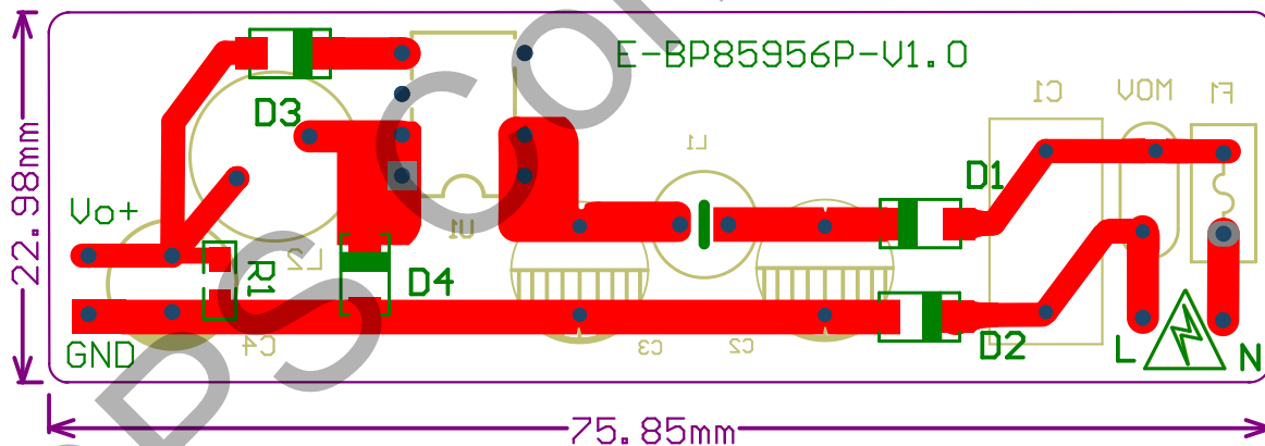
图 14. BP85956P 设计实例,PCB Layout (单面板)
