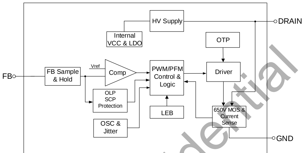
图 4. BP85956P 内部框图
