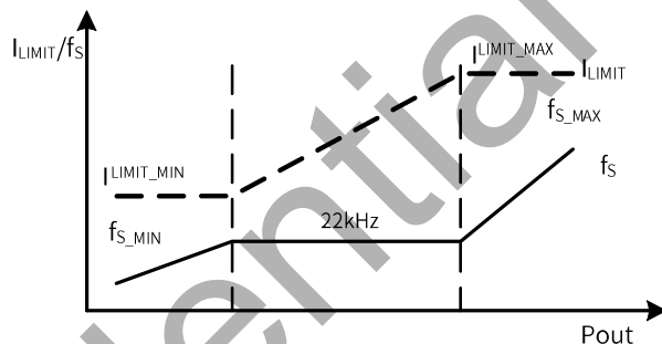
图 8. 控制模式
