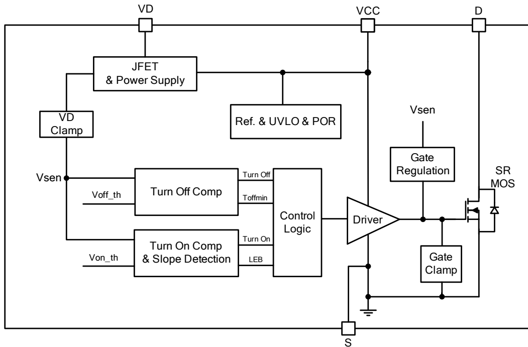
图 3. BP6211BS 内部框图
