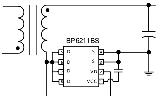
图 1. BP6211BS 典型应用电路
