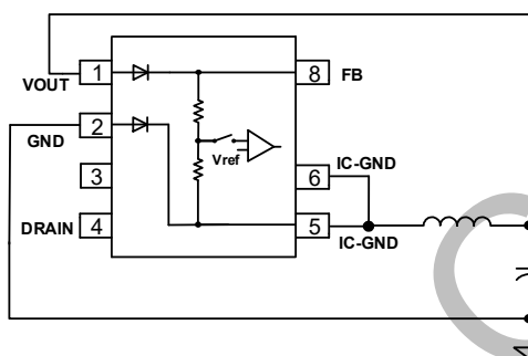
图 7. 输出电压采样示意图
