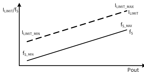
图 8. 控制模式
