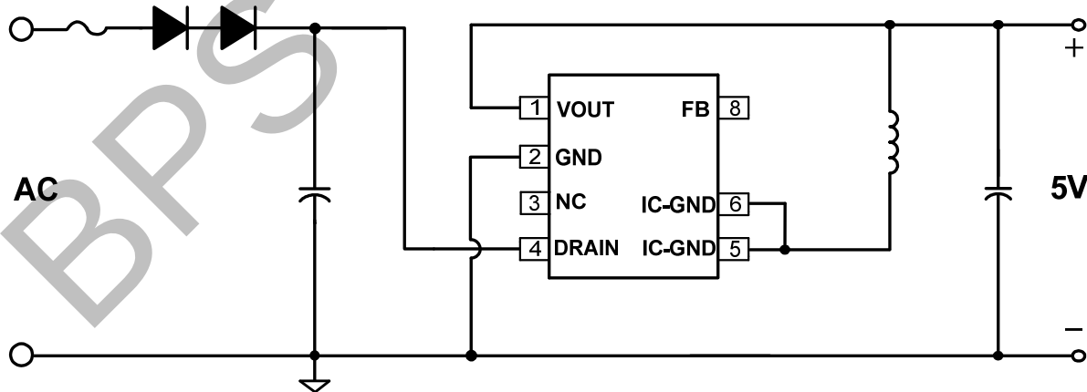
图 1. BP85222D 典型 Buck 应用电路
