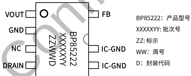
图 3. 管脚封装图
