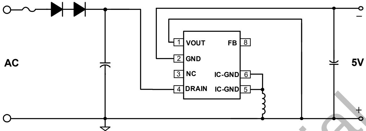
图 2. BP85222D 典型 Buck-Boost 应用电路
