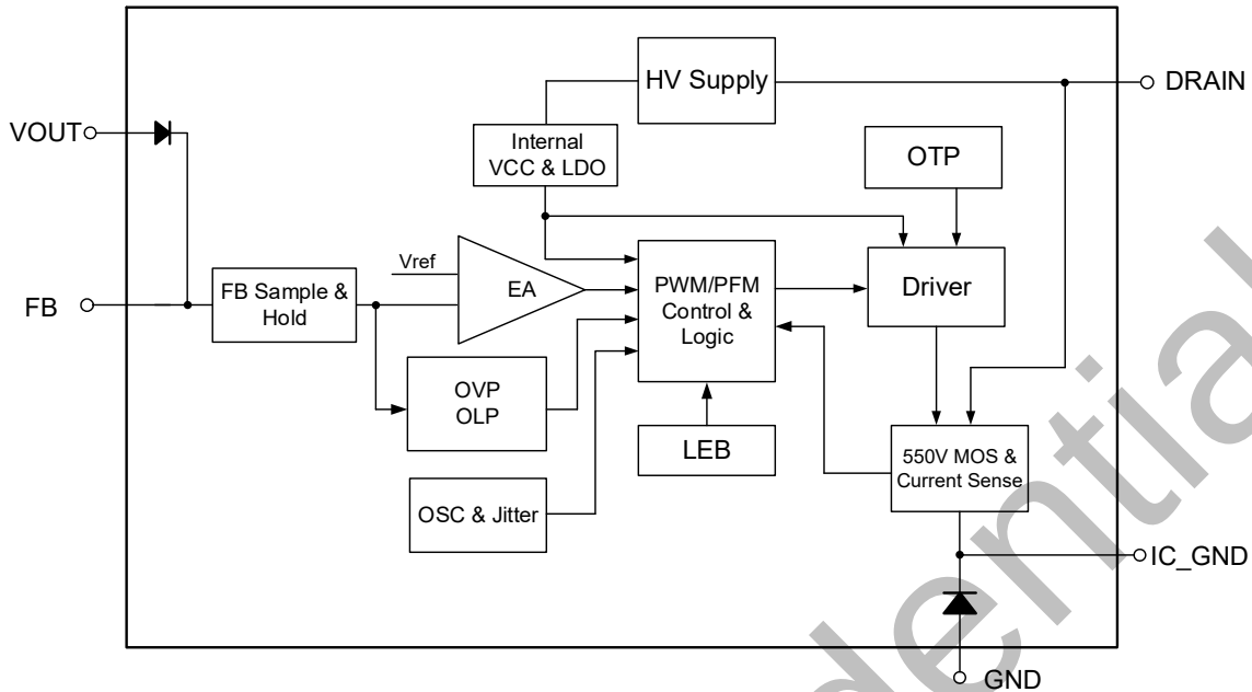
图 4. BP85222D 内部框图
