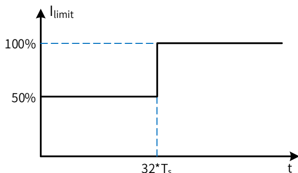
图 6. 软启动过程
