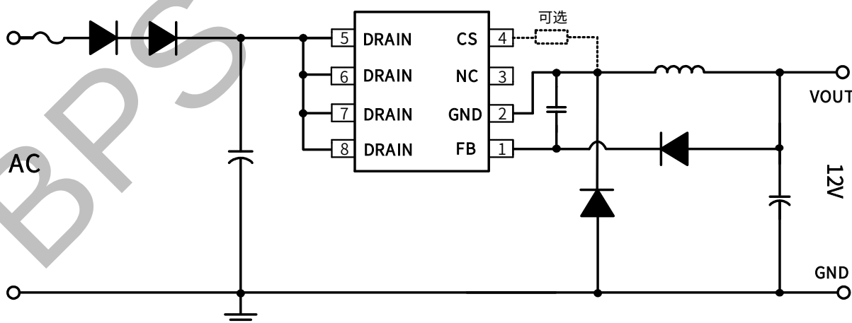
图 1. BP85958D 典型 BUCK 应用电路
