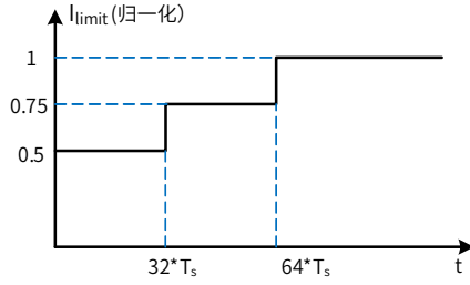
图 5. 软启动过程
