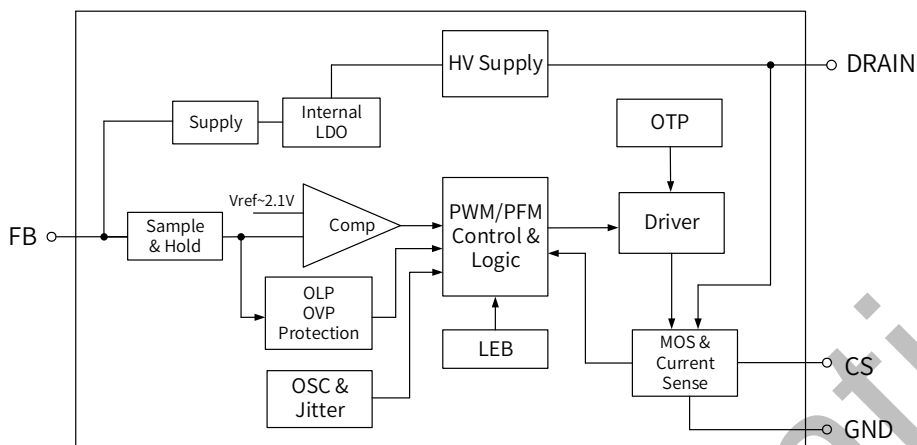
图 3. BP85958D 内部框图
