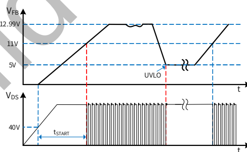
图 4. 高压启动与 FB 欠压保护时序
