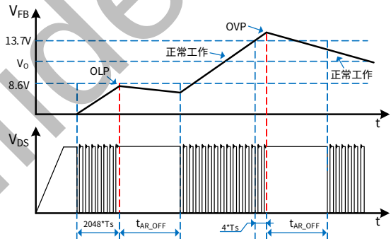
图 7 过载保护、输出过压保护工作模式
