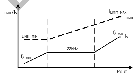
图 6. 控制模式
