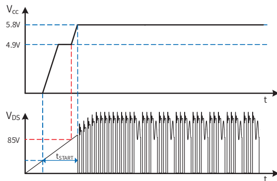
图 5. 高压启动时序
