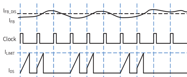
图 9. 脉冲数控制
