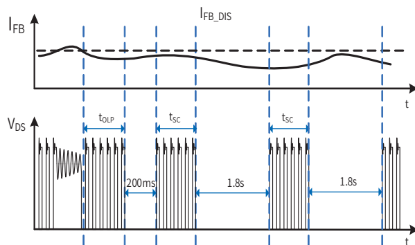
图 10. 故障保护与自动重启时序
