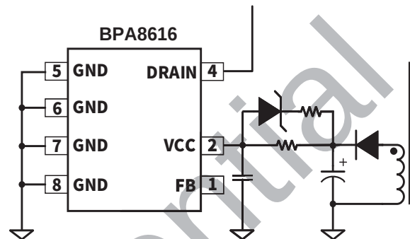
图 7. VCC 引脚实现输出电压保护
