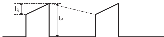
图14. 连续模式下初级电流波形
