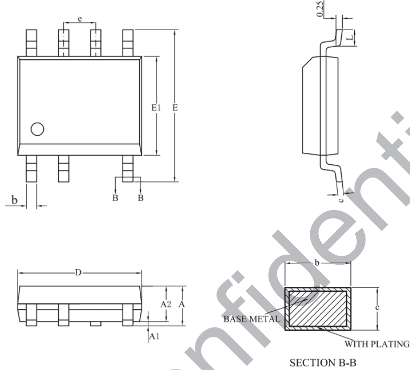
SOP-7 封装外形尺寸
