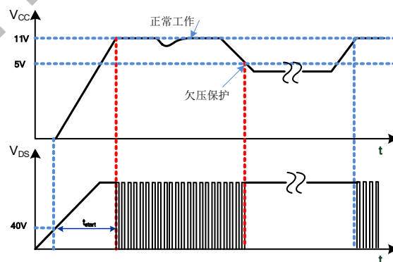
图 4. 高压启动与 VCC 欠压保护时序
