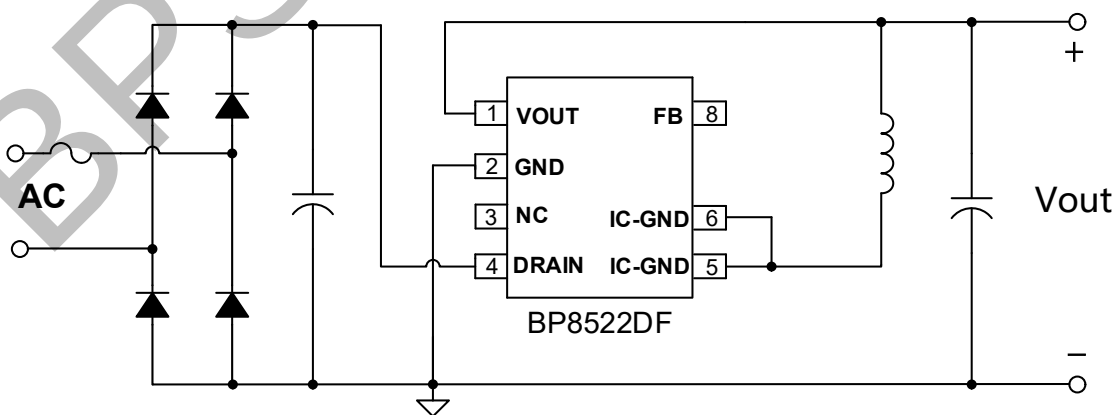
图 1. BP8522DF 典型 Buck 应用电路
