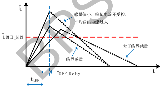
图 11. 空载下的电感电流
