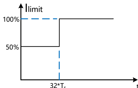
图 5. 软启动过程
