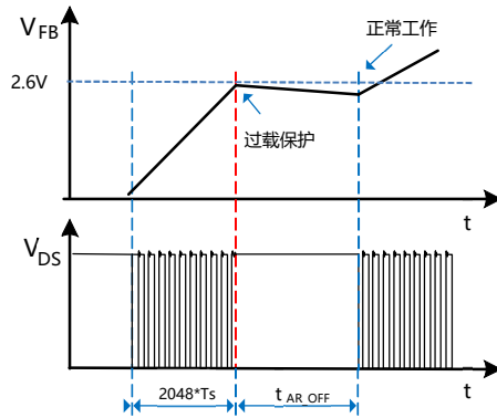
图 8 过载保护工作模式
