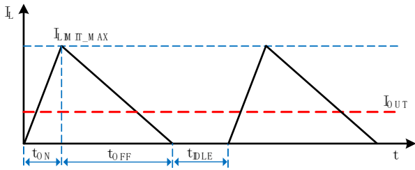
图 10. DCM 模式下的电感电流
