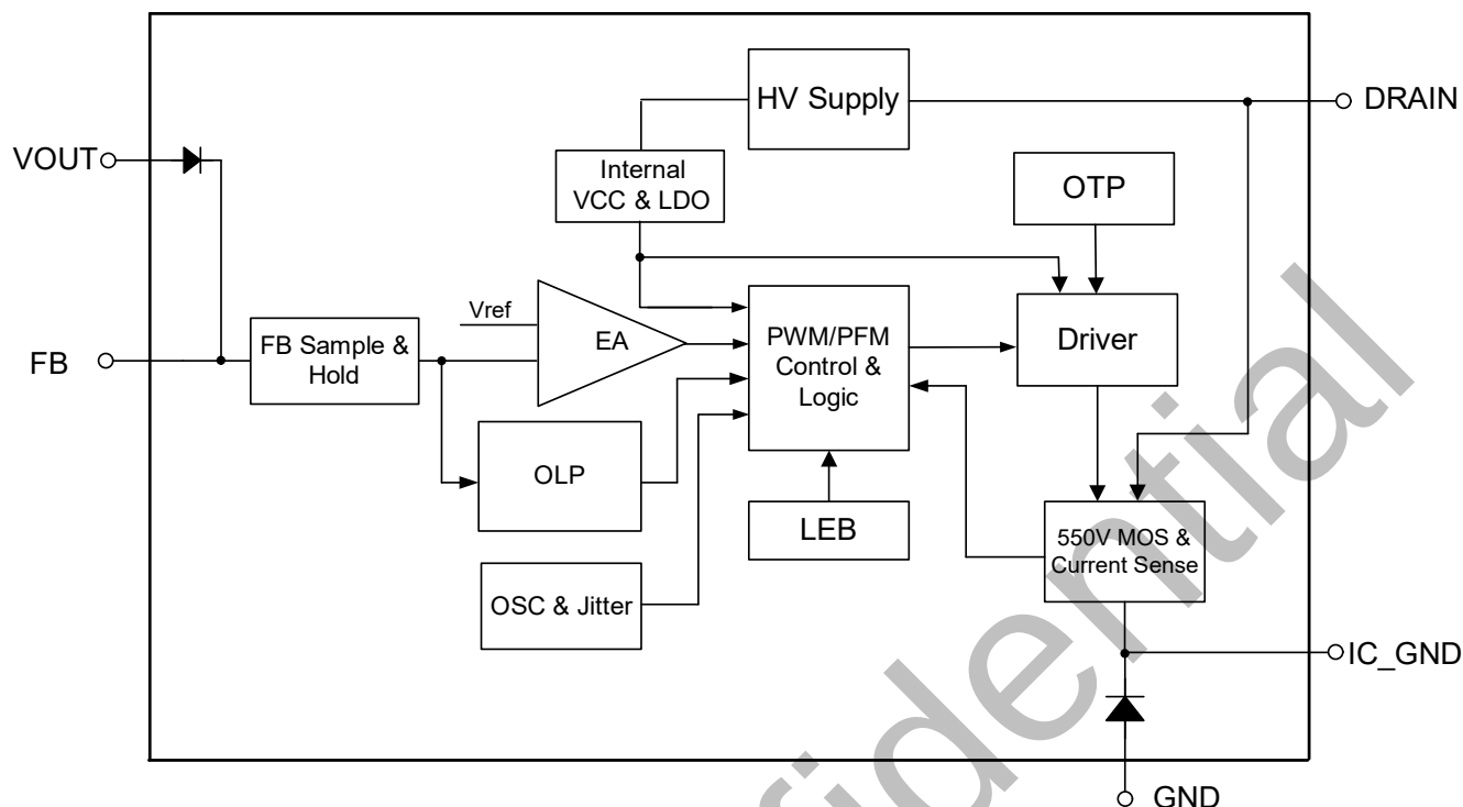
图 3. BP8522DF 内部框图
