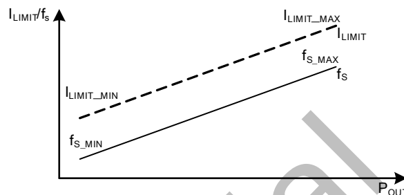
图 7. 控制模式
