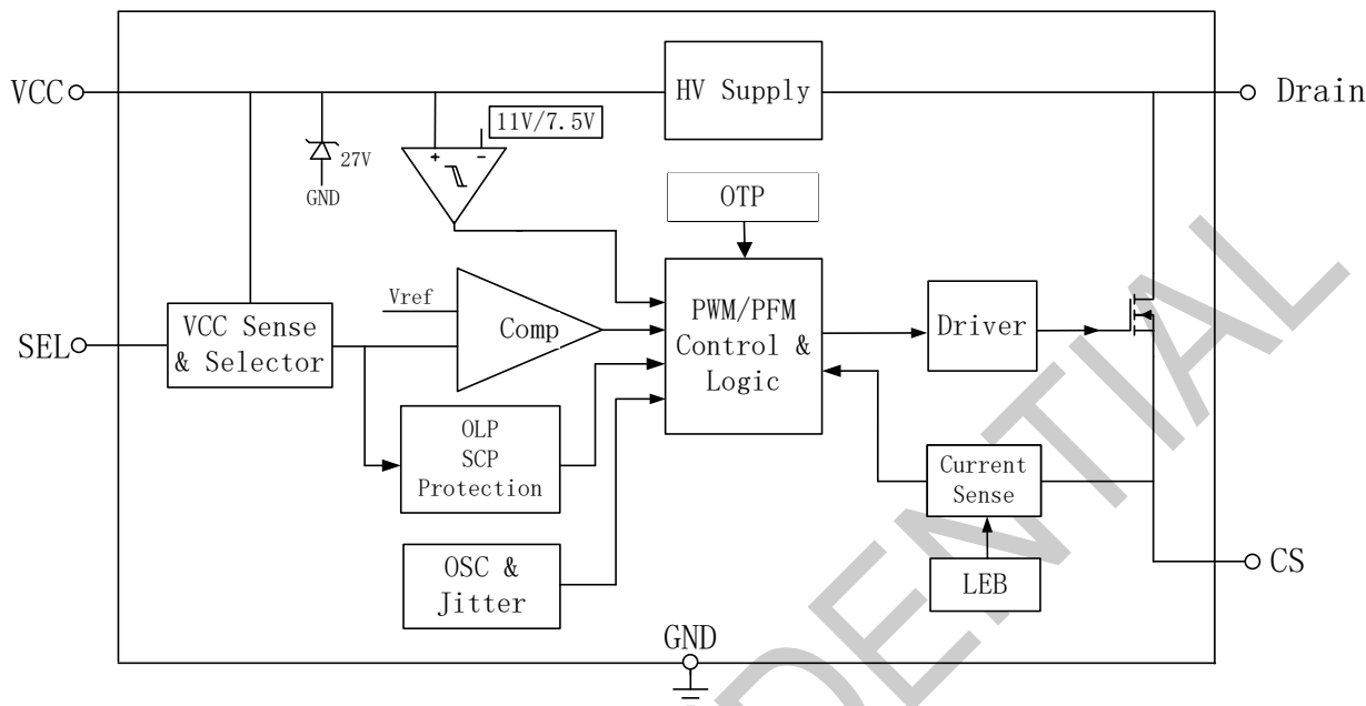
图 4 BP2523X 内部框图
