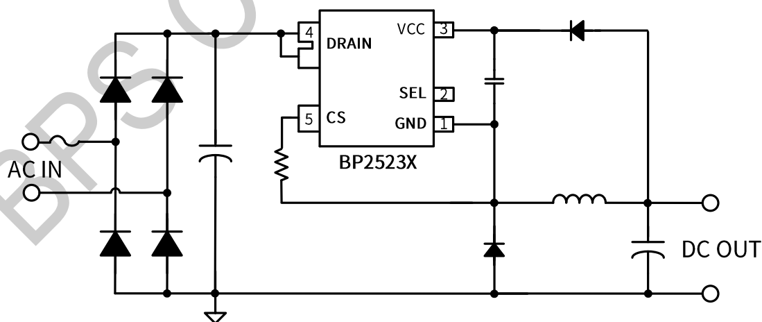
图 1 BP2523X 典型应用
