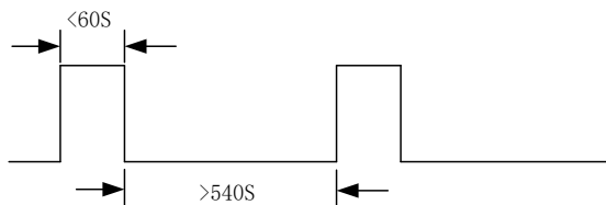
图 3 瞬时脉冲示意图
