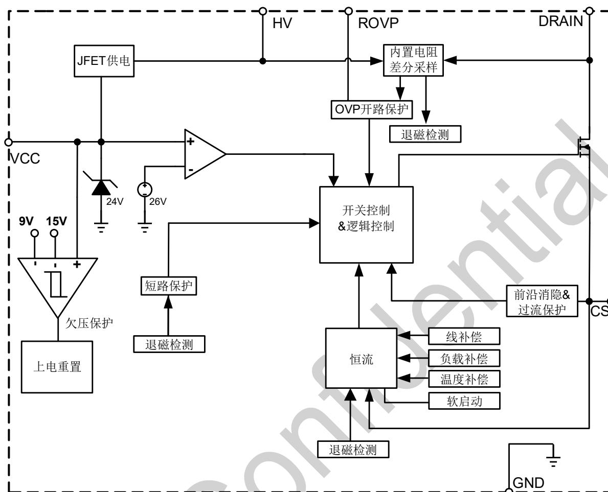
图 3 BP3186DB 内部框图
