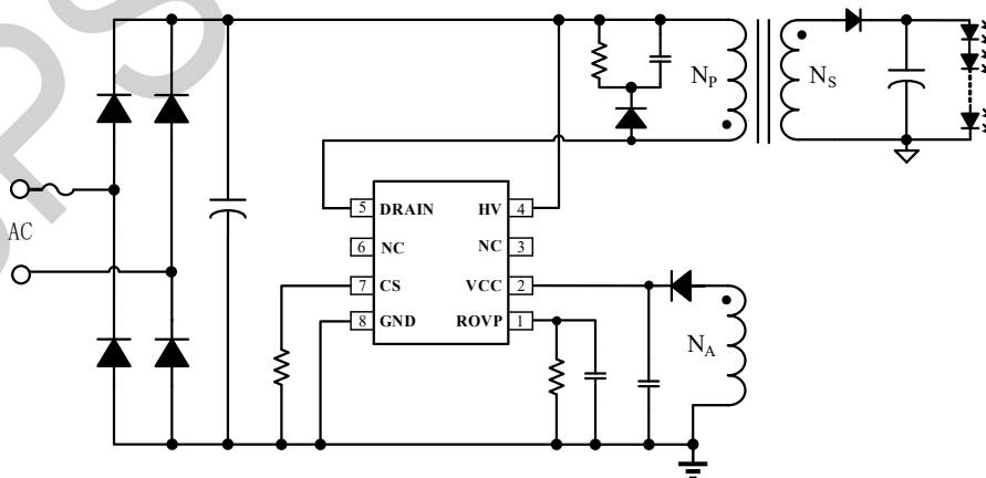
图 1 BP3186DB 典型应用电路
