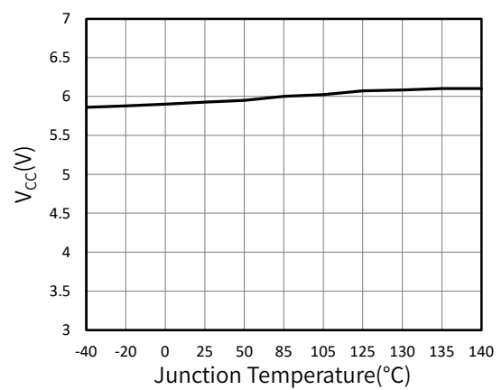
图 21. V CC vs. Temperature
