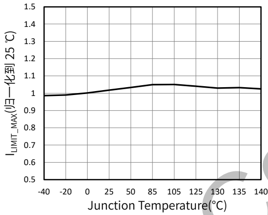
图 18. I LIMIT_MAX vs. Temperature
