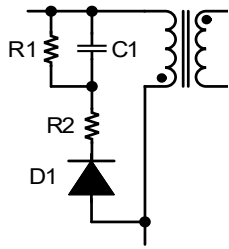
图14. RCD钳位电路
