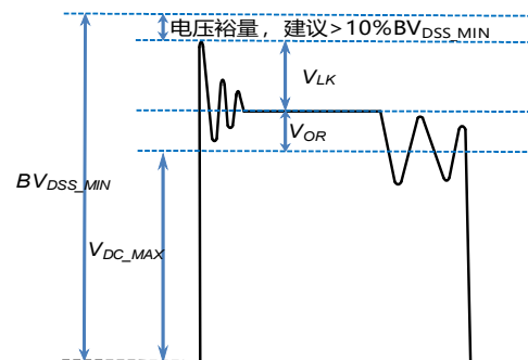
图11. MOSFET漏极电压波形
