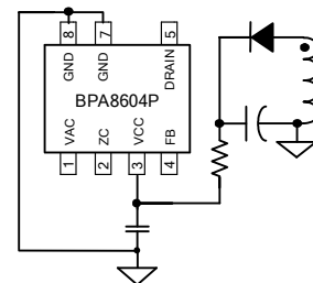
图 13. 辅助绕组供电电路
