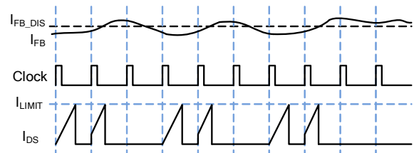
图 8. 脉冲数控制
