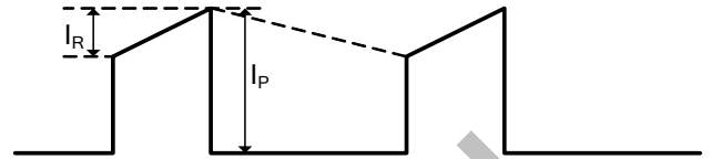
图12. 连续模式下初级电流波形
