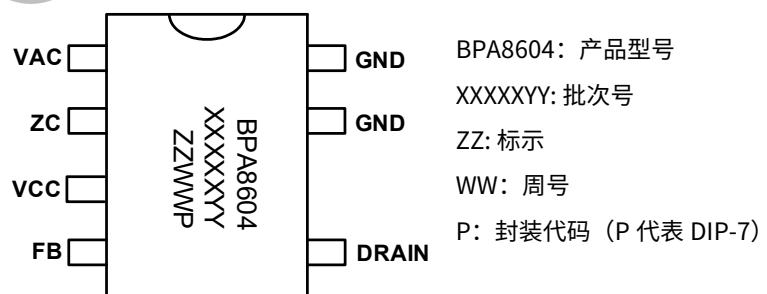
图 3. DIP-7 管脚封装图
