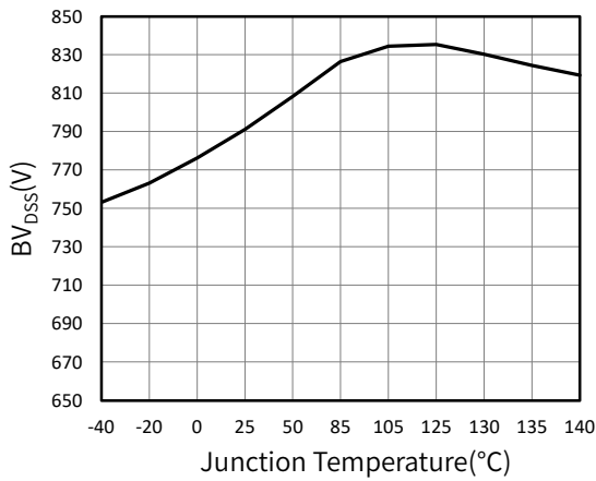
图 16. BV DSS vs. Temperature
