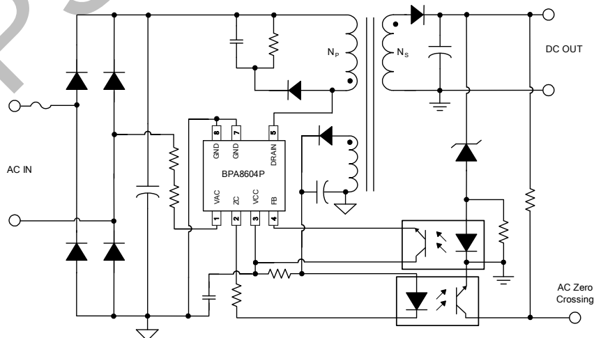
图 1. BPA8604P 过零检测典型应用电路
