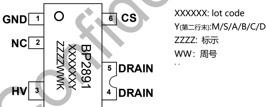
图 2 管脚封装图
