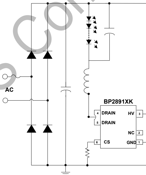
图 1 BP2891XK 典型应用图
