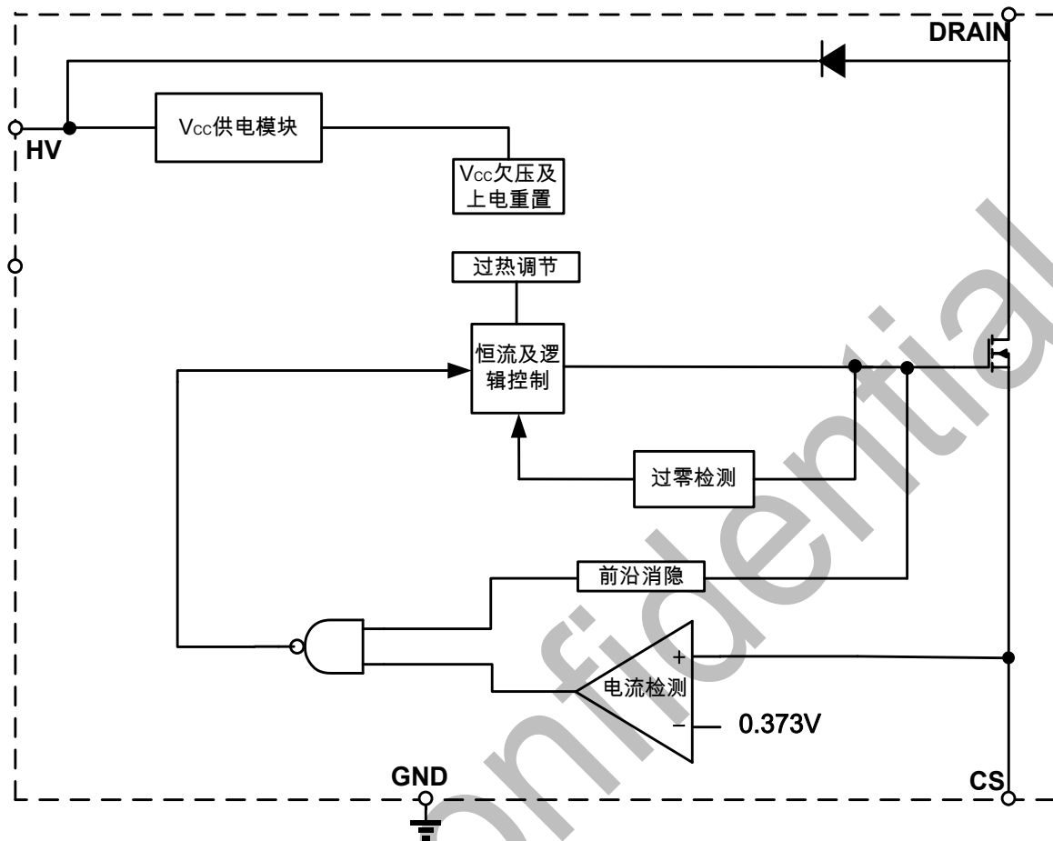
图 3 BP2891XK 内部框图
