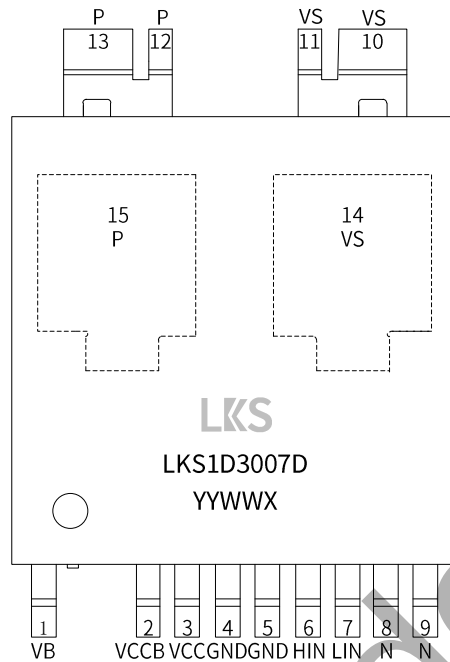
图 2. LKS1D3007D 管脚封装图
