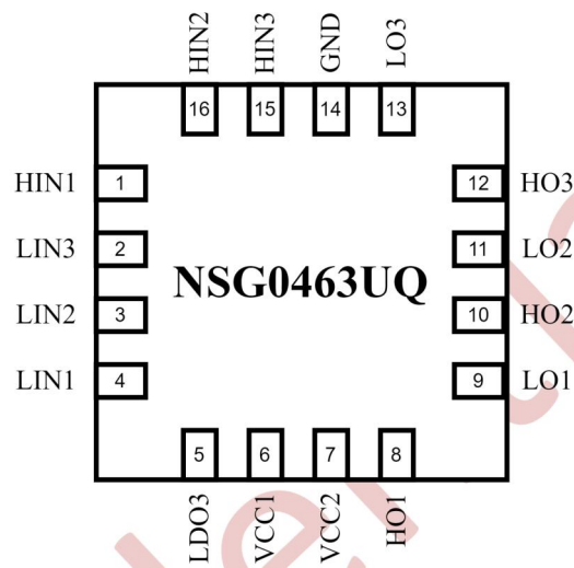
图 6-1 16-脚 QFN 顶视图
