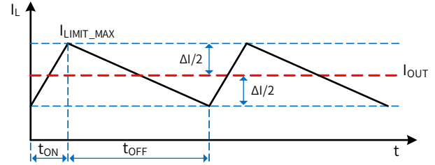
图 8. CCM 模式下的电感电流
