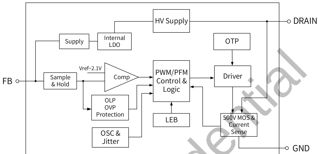
图 3. BP85957DL 内部框图
