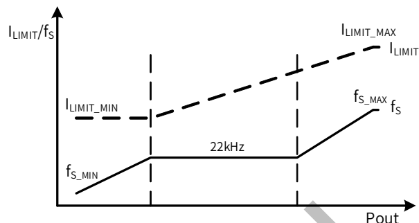
图 6. 控制模式
