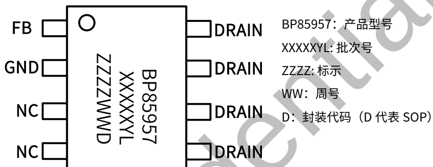
图 2. 管脚封装图
