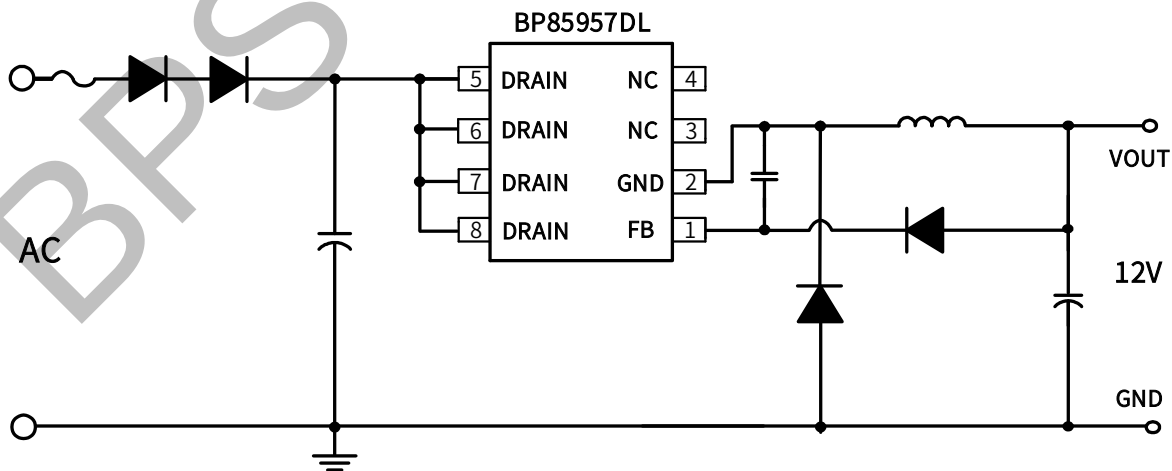
图 1. BP85957DL 典型 BUCK 应用电路
