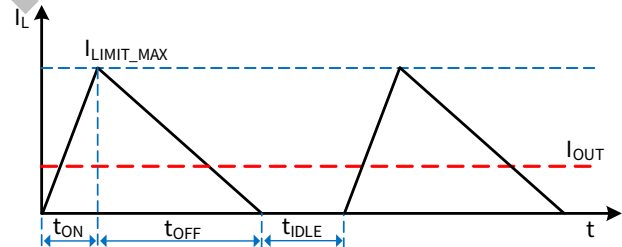
图 9. DCM 模式下的电感电流
