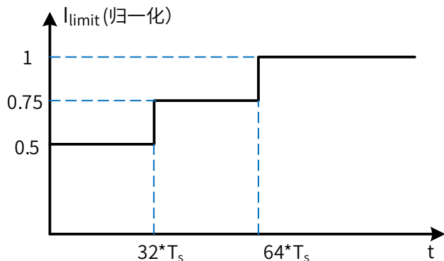
图 5. 软启动过程
