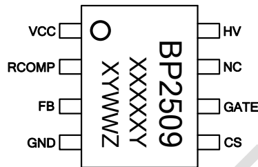
图 2 管脚封装图
