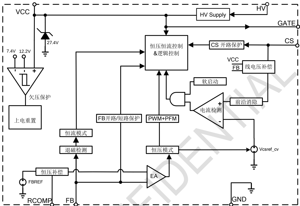
图 3 BP2509 内部框图
