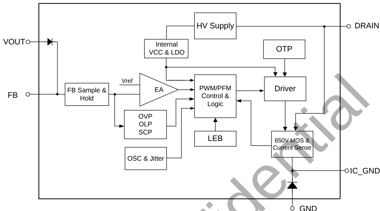
图 4. BP85226DF 内部框图
