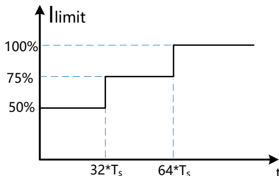
图 6. 软启动过程
