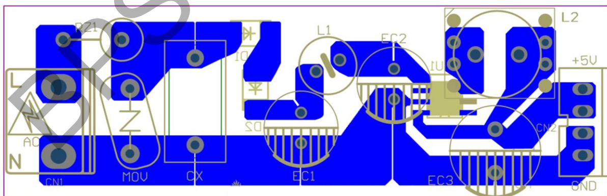
图 14. BP85226DF 设计实例 PCB Layout (单面板)
