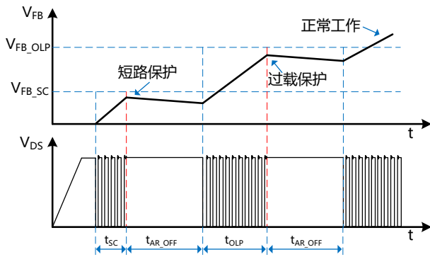
图 9. 短路保护、过载保护工作模式
