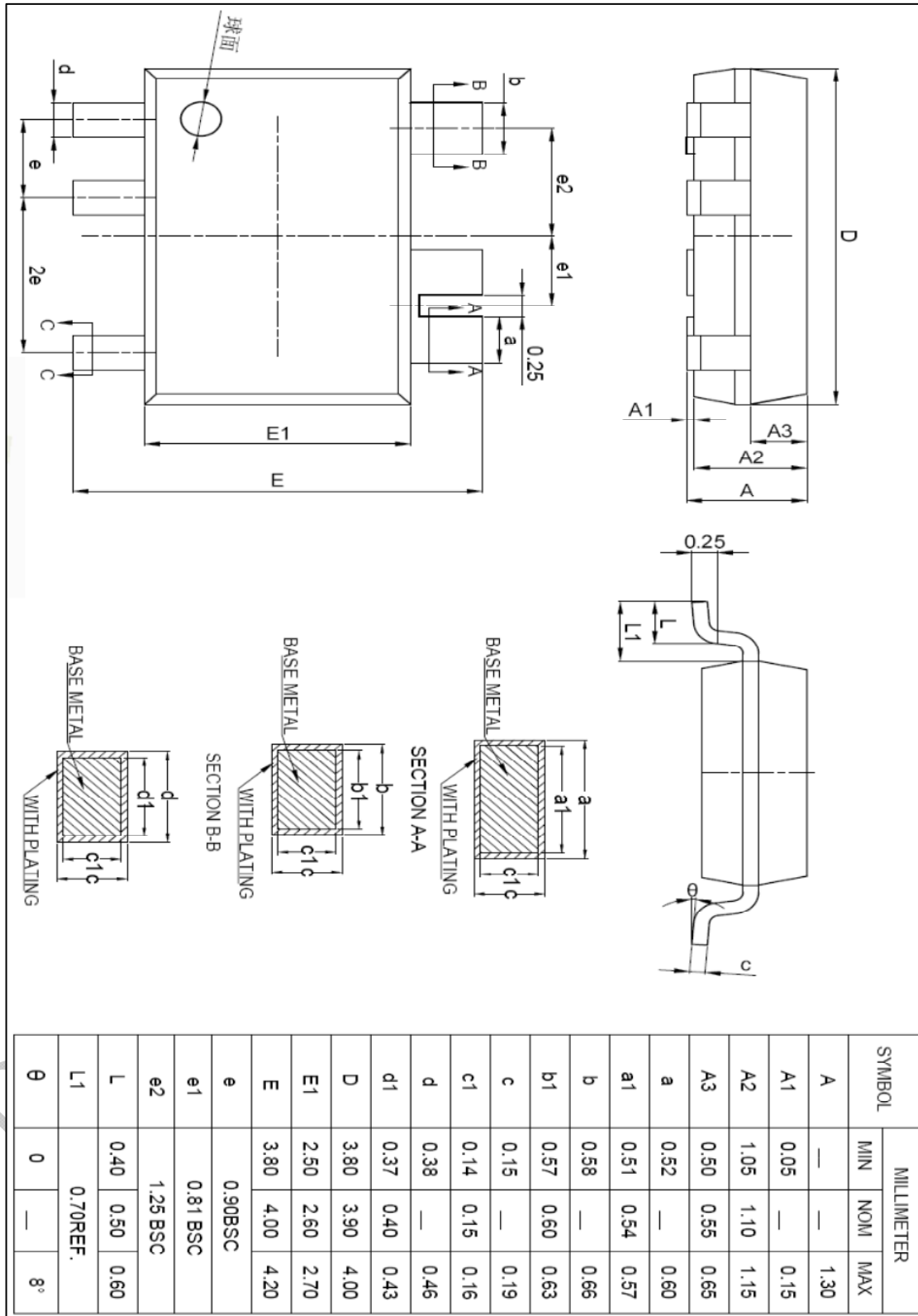
SOT33-5A 封装外形尺寸
