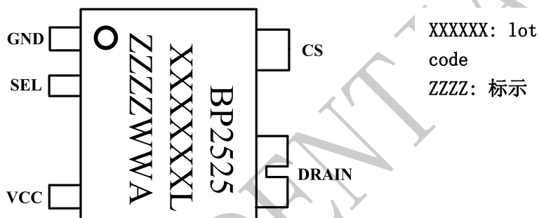
图 2 管脚封装图
