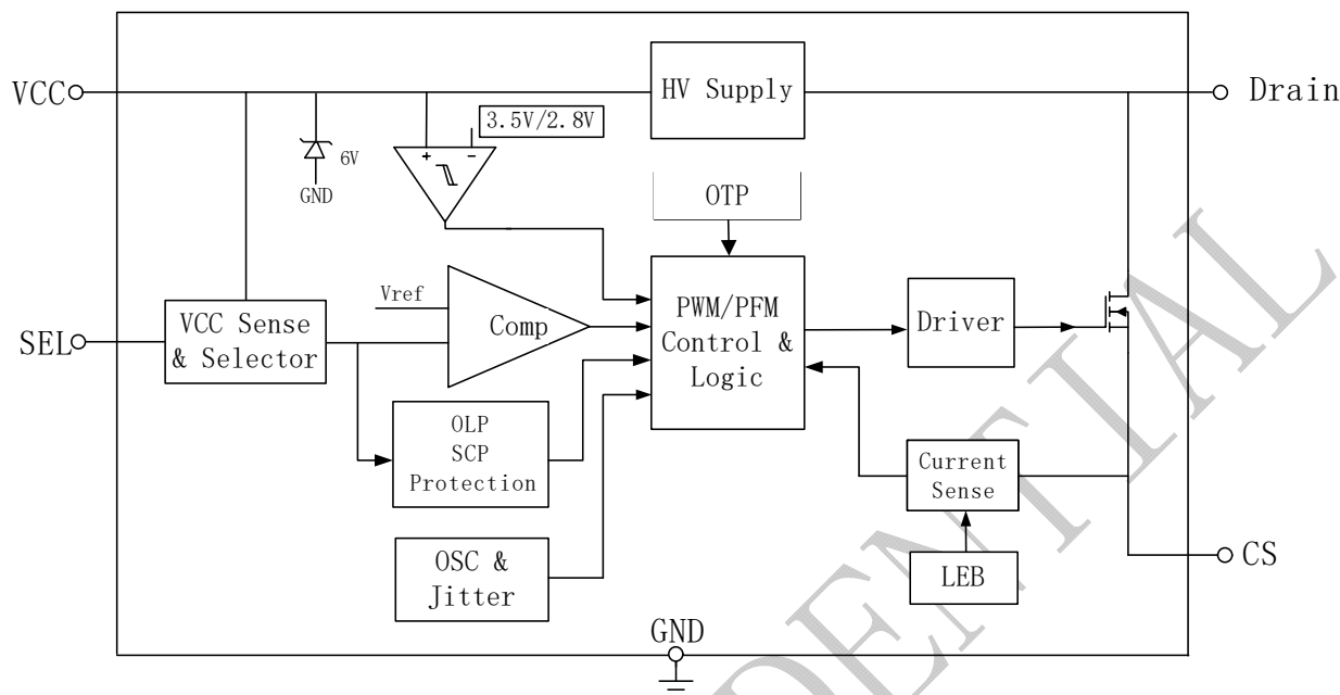
图 4 BP2525AHL 内部框图
