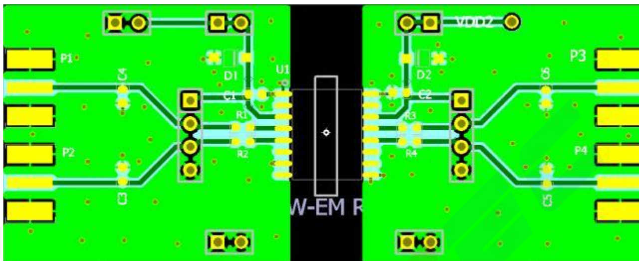
图 8. 推荐 PCB 布局
