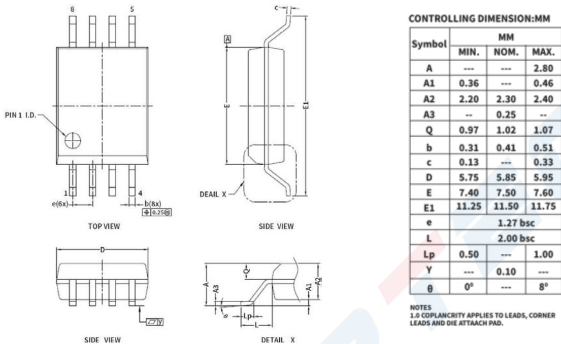
图 20. ISO772X SOW8L 封装
