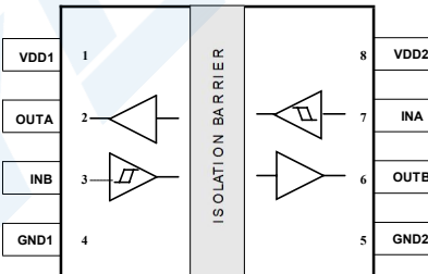
图 5. ISO7721NX / ISO7721GX 管脚
