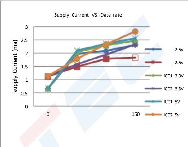
图 12. 电源电流 vs. 数据率 T_A=25^{\circ}\text{C} C_L=\text{No Load}
