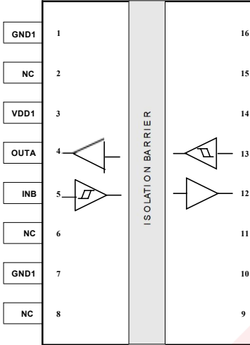
图 2. ISO7721WX 管脚
