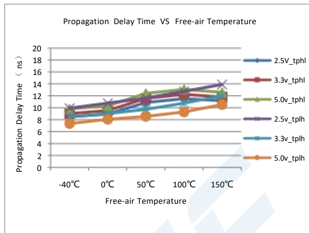
图 16. 传播延时 vs. 大气温度
