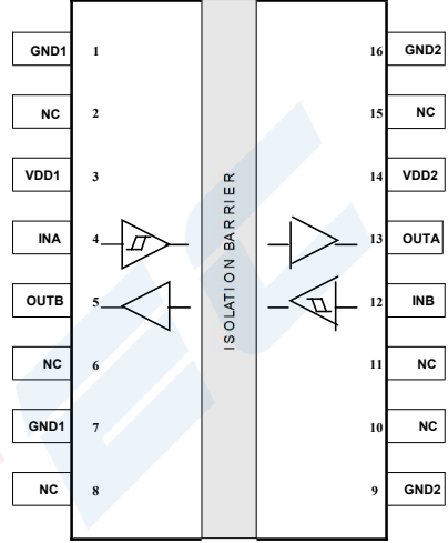
图 3. ISO7722WX 管脚
