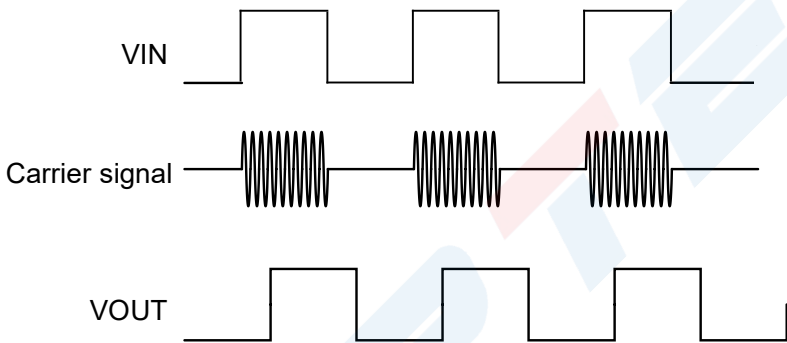
图 17. OOK 调制机制
