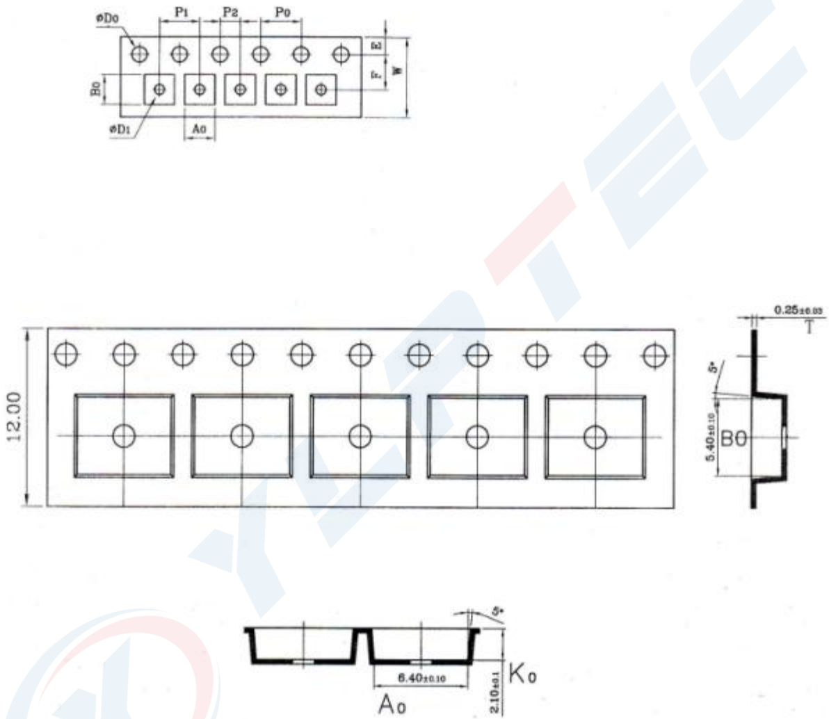
图 26.ISO772X NB SOIC-8 编带信息
