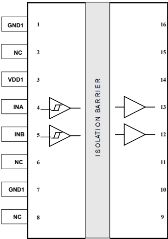
图 1. ISO7720WX 管脚
