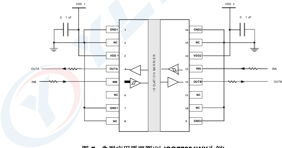
图 7. 典型应用原理图(以 ISO77221WX为例)
