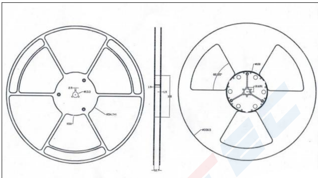
图 25. ISO772X NB SOIC-8 卷带信息
