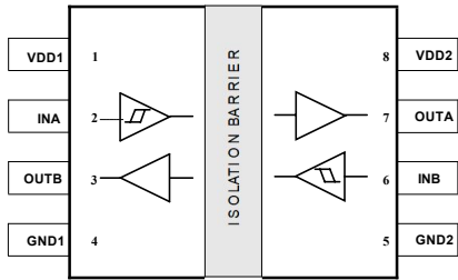
图 6. ISO7722NX / ISO7722GX 管脚
