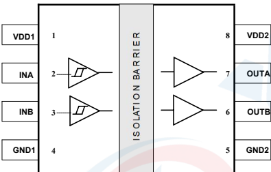
图 4. ISO7720NX / ISO7720GX 管脚
