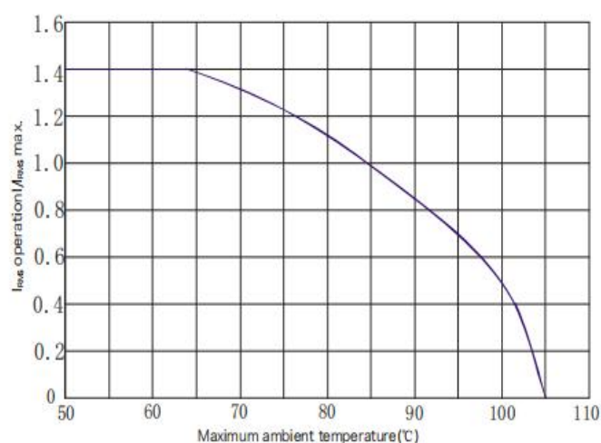
纹波电流降额曲线
