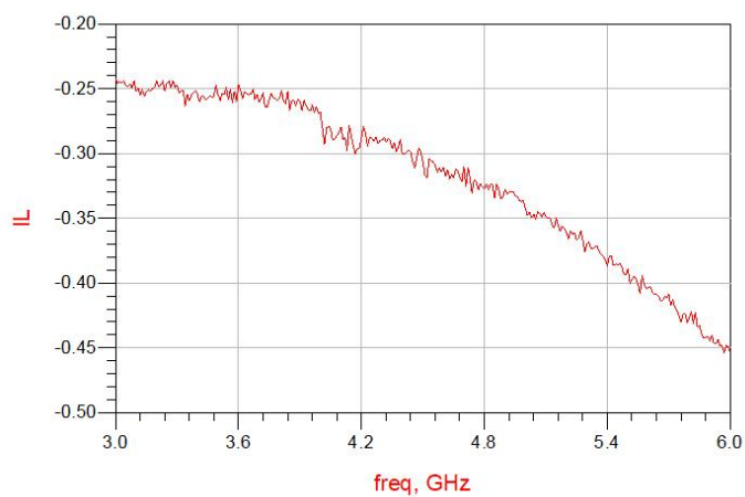
Figure 10. MHC58S03 IL
