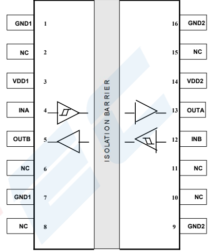
图 3. ISO7722WX 管脚
