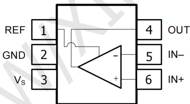
SC70-6(SOT-363)
