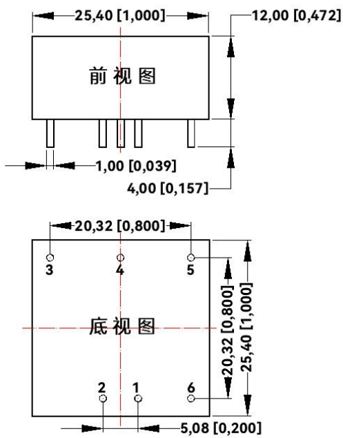
URB2405YMD-15WR3 尺寸图
