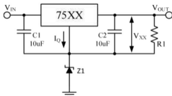
图 7 提高输出电压电路 2
