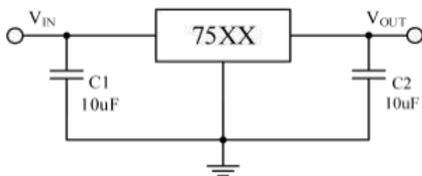
图 3 基本电路
