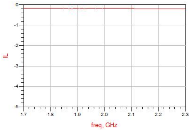
Figure 11. MHC21X03 IL
