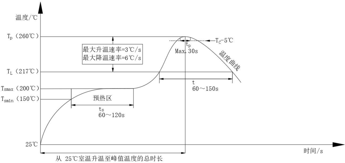
再流焊过程示意图
