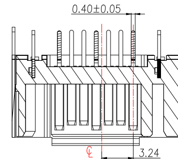
剖面 B-B
