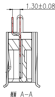
剖面 A-A
