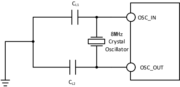
图 4-5 外接 8M 晶体典型电路
