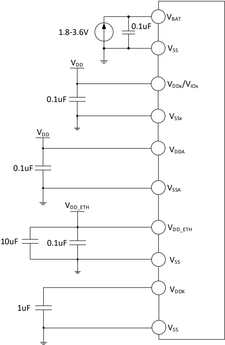
图 4-1-2 CH32V317 常规供电典型电路
