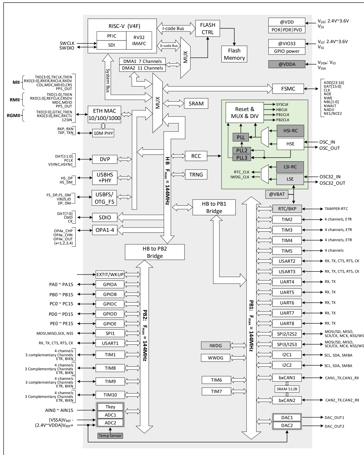
图 2-1-1 CH32V303/305/307 系统框图
