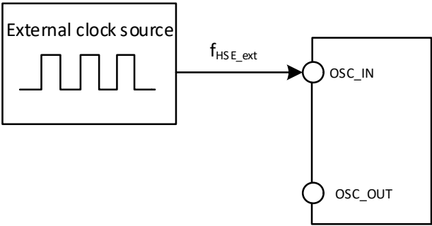
图 4-3 外部提供高频时钟源电路
