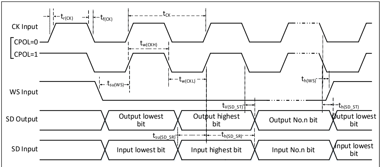
图 4-13 I2S 总线从模式时序图
