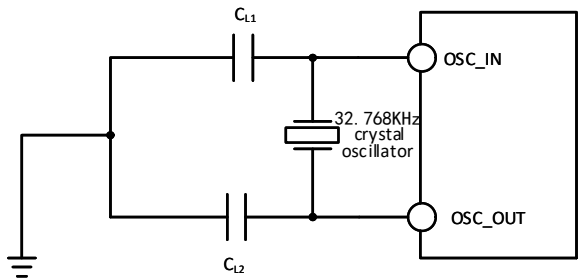
图 4-6 外接 32.768\text{K} 晶体典型电路
