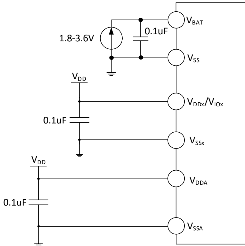
图 4-1-1 CH32V303/305/307 常规供电典型电路
