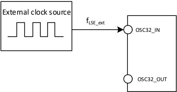
图 4-4 外部提供低频时钟源电路
