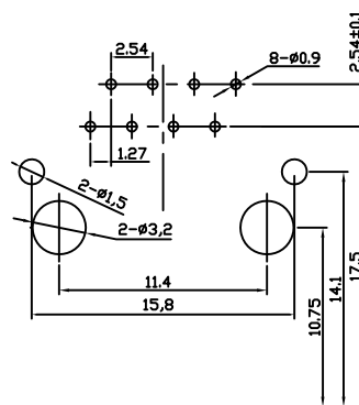
P. C. B参考图
